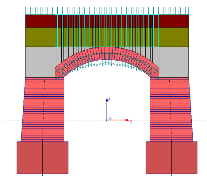
Fig. 2.1.23. Carichi per CCE n.2
