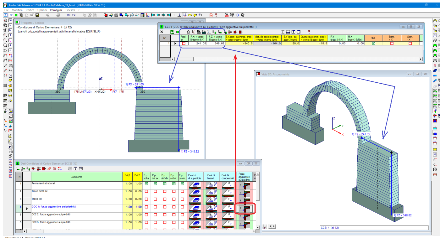
Fig. 2.3.25. CCE aggiuntive create dall'importazione delle azioni di interscambio, con focus sulla CCE n°4
