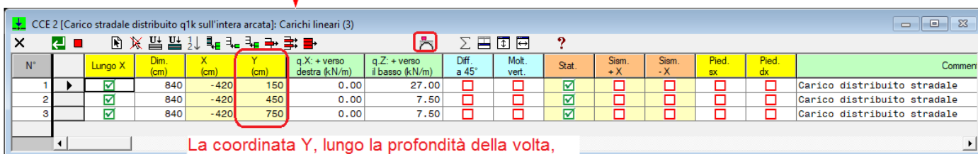
Fig. 2.5.6. Carichi distribuiti da ponte stradale
