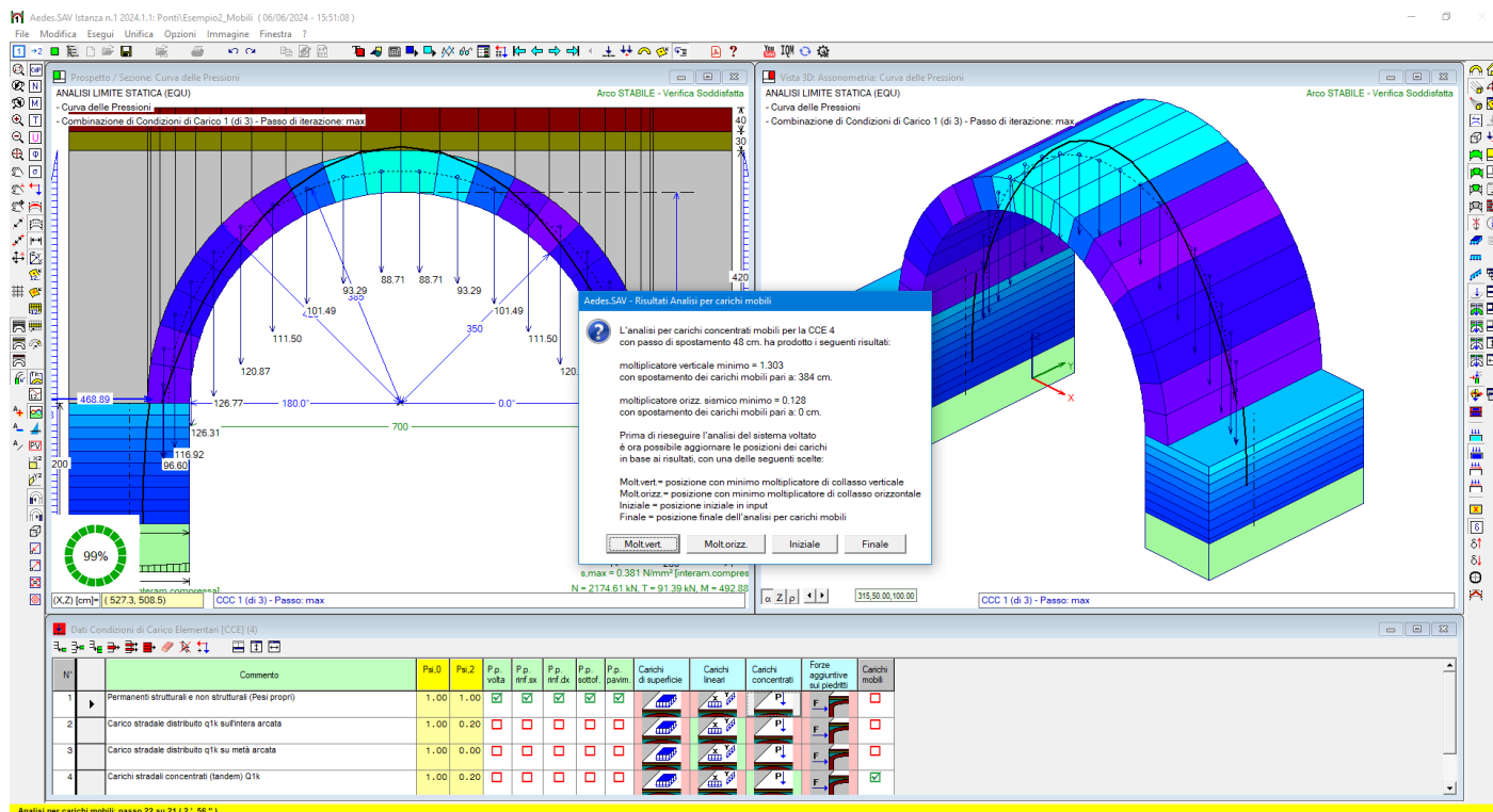
Fig. 4.3.2. Termine dell'analisi per carichi mobili
