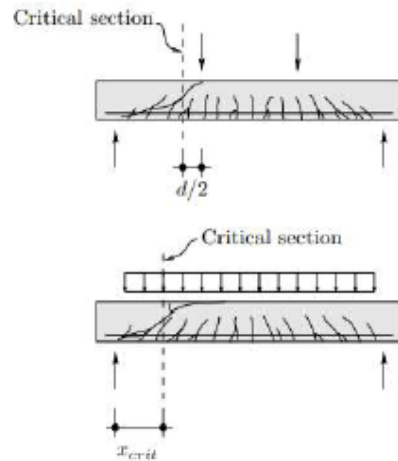
Figura 14-4: Fessura critica a taglio [21]
