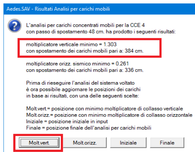
Fig. 2.2.10. Report dell'analisi per carichi mobili
