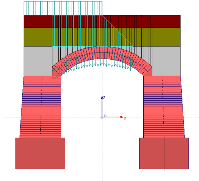
Fig. 2.1.24. Carichi per CCE n.3
