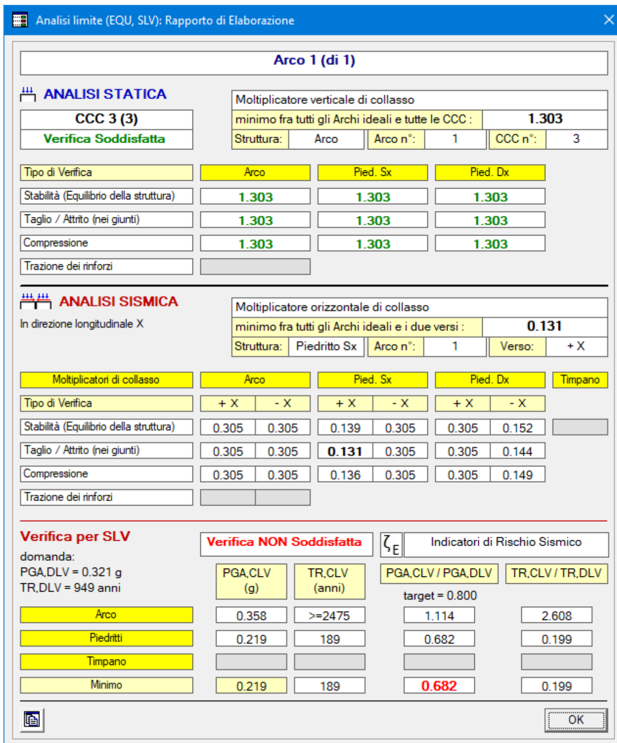
Fig. 2.2.15. Analisi del ponte per viabilità standard
