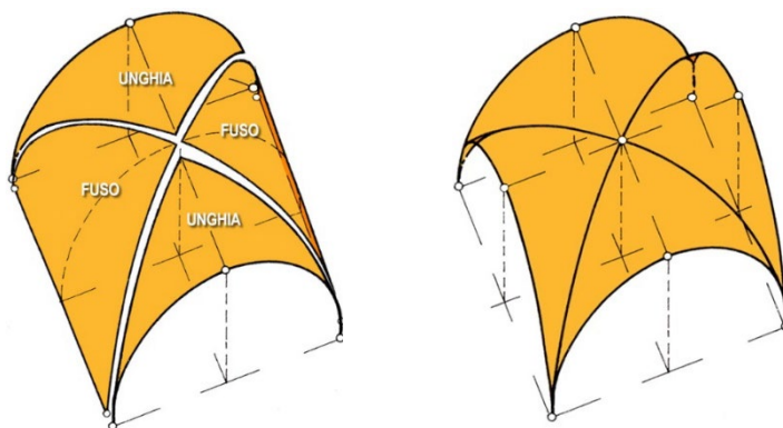
Fig. 1.3.1. (a) Fusi e unghie di una volta a botte. (b) Volta a crociera ottenuta dalla composizione di 4 fusi (immagini tratte da didatticarte.it)
