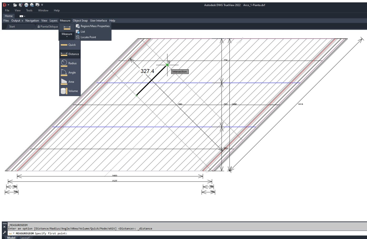
Fig. 2.4.17. Misura precisa della fascia che schematizza la volta retta circolare
