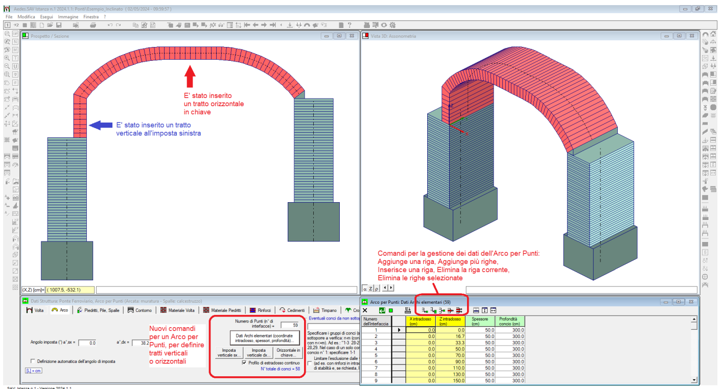
Fig. 1.4.8. Inserimento di porzioni verticali e/o orizzontali in un arco per punti
