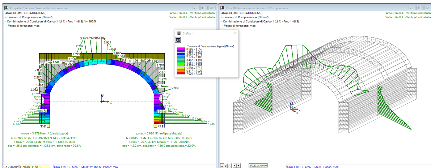
Fig. 2.4.30. Tensioni di compressione
