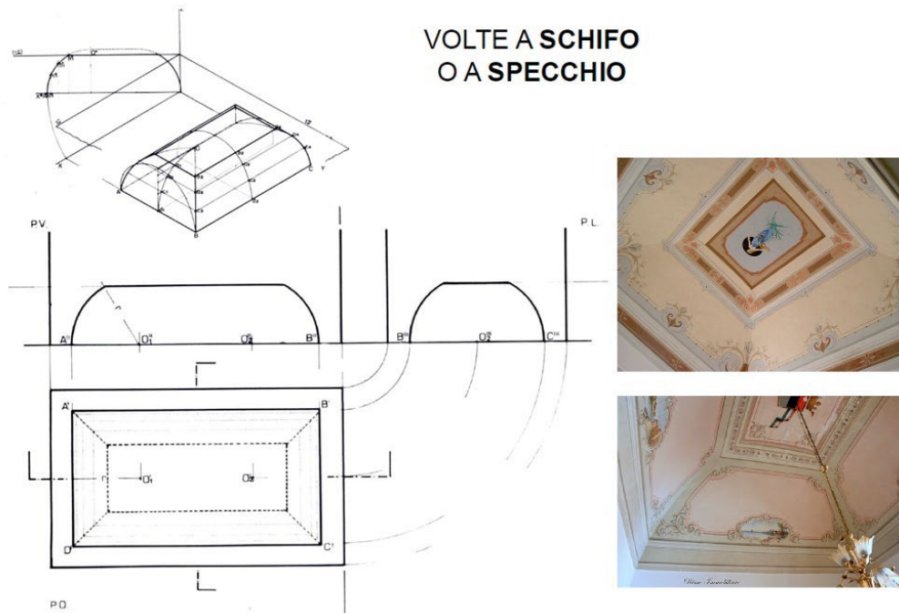
Fig. 1.4.10. Volta a schifo
