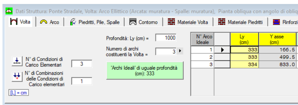
Fig. 2.4.10. Profondità della volta e suddivisione, se non è arco singolo, in archi ideali affiancati
