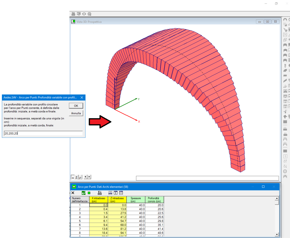
Fig. 1.4.3. Profondità variabile per l'arco per punti
