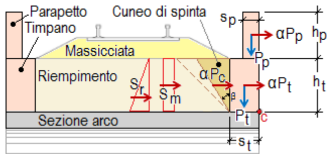
Fig. 2.1.17. Geometria del timpano e azioni verticali e orizzontali
