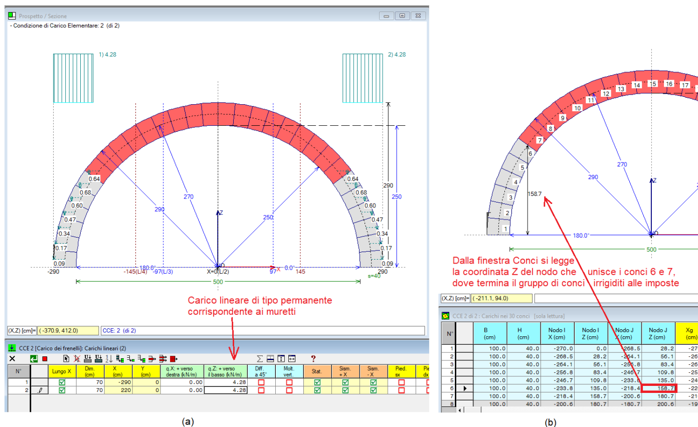
Fig. 1.6.3.3. Input dei carichi corrispondenti al peso dei muretti (frenelli)
