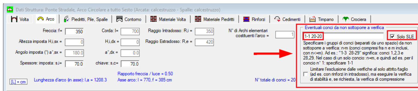
Fig. 3.4.6. Esclusione dalle verifiche dei conci iniziale e finale per il modello elastico
