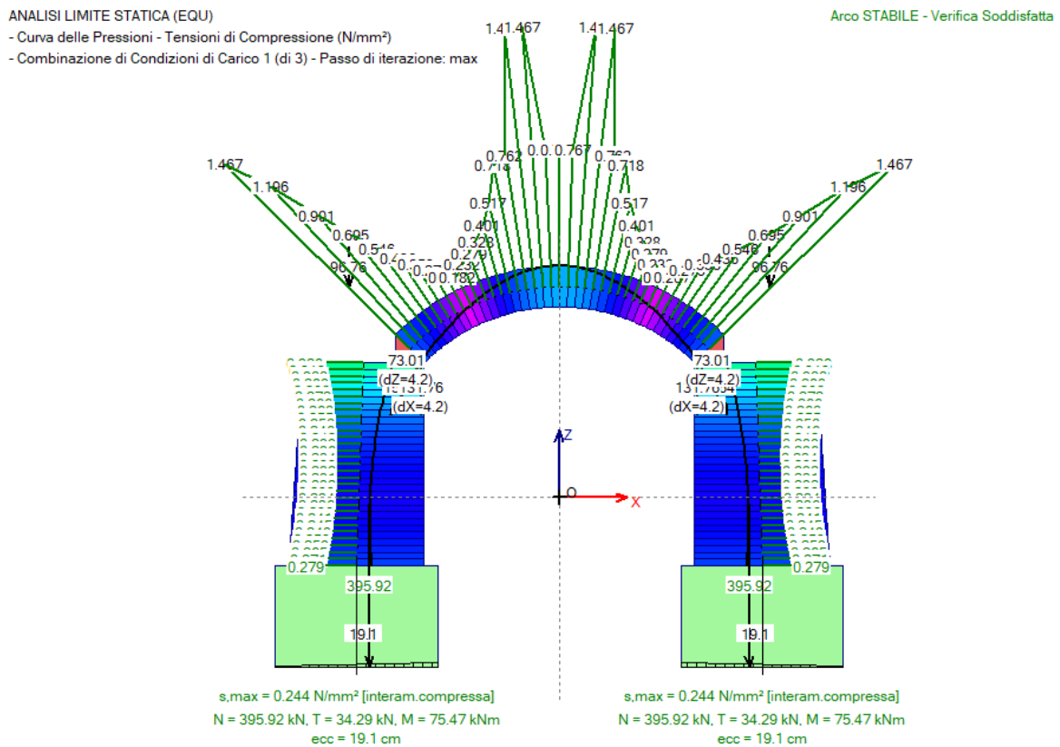
Fig. 2.1.41. Risultati Stato di Progetto, Analisi Statica, CCC 3. Curva delle pressioni e Tensioni di Compressione
