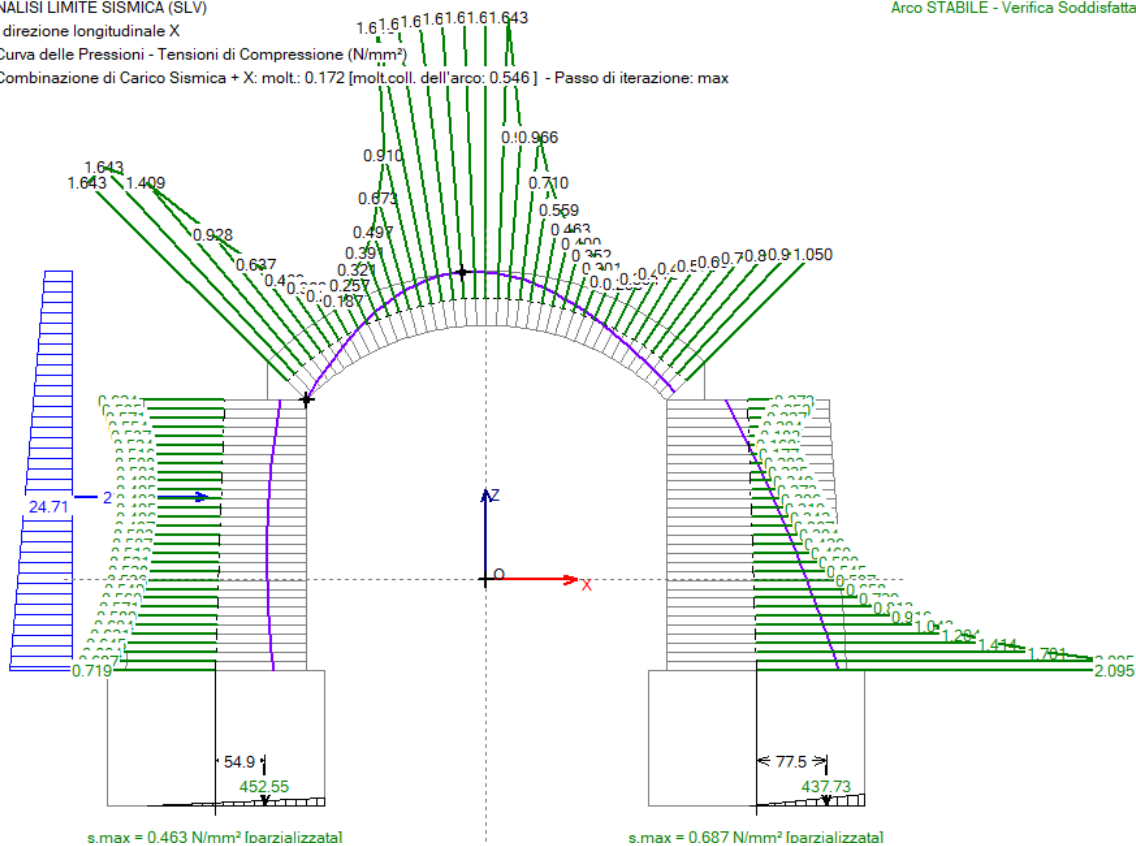
Fig. 2.1.37. Risultati Stato Attuale, Analisi Sismica +X. Tensioni di Compressione
