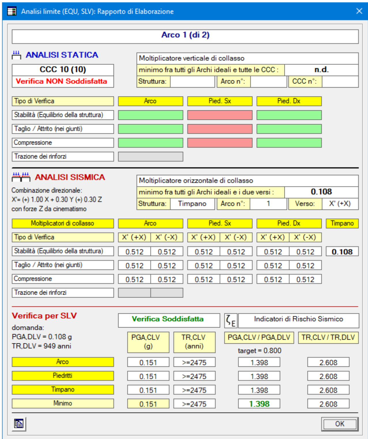
Fig. 2.3.57. Campata intermedia: risultati definitivi
