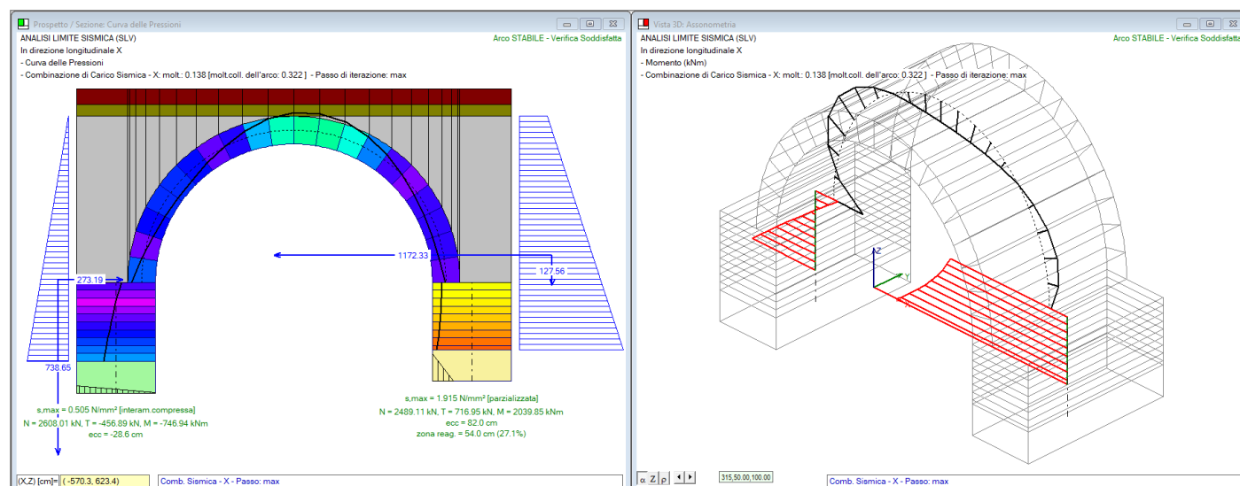
Fig. 2.2.14. Verifica sismica in direzione +X
