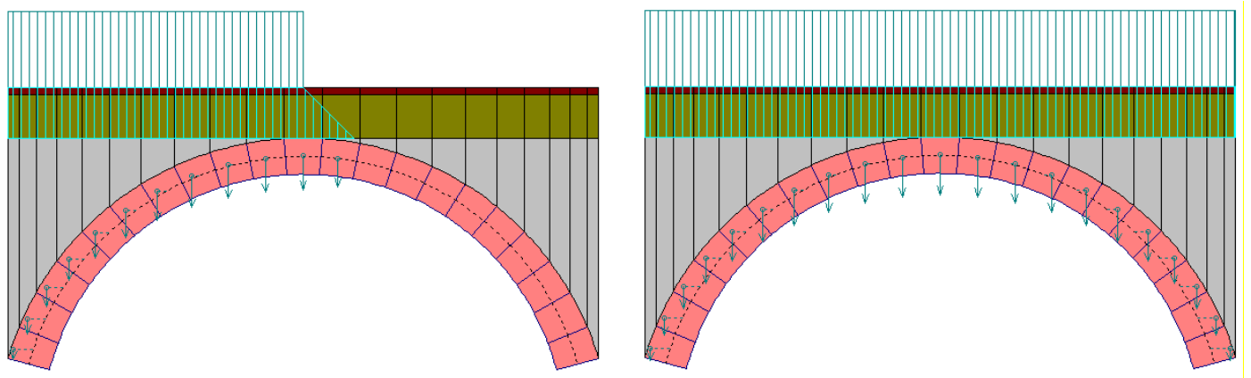
Fig. 4.1.4. Carichi distribuiti parziali o uniformi
