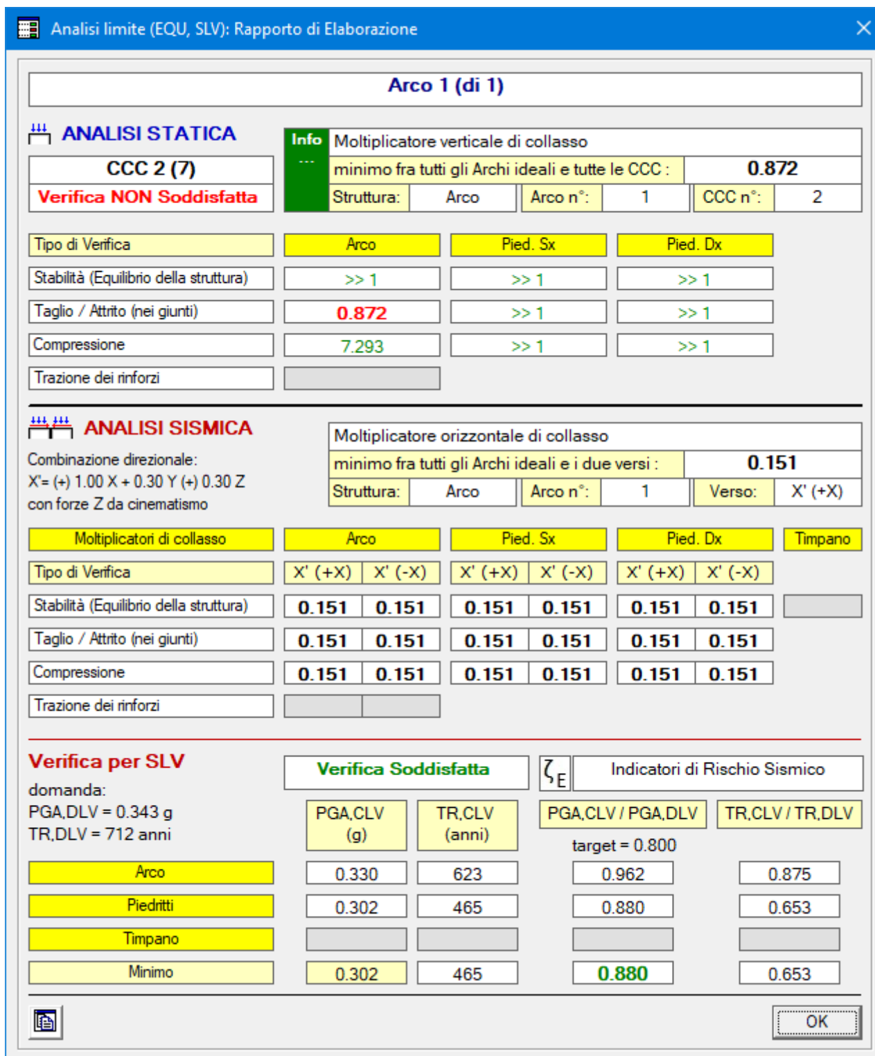
Fig. 2.3.12. Campata SX: risultati per la fase 1
