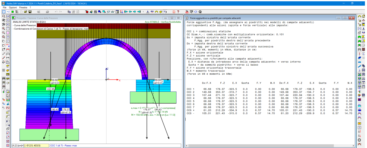
Fig. 2.3.21. Campata DX: quadro riepilogativo forze alle imposte (aggiuntive per la campata C1)
