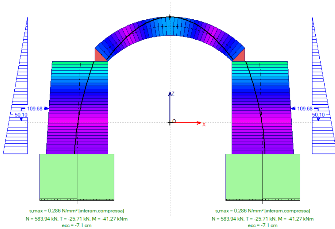
Fig. 2.1.33. Risultati Stato Attuale, Analisi Statica, CCC 3. Curva delle pressioni
