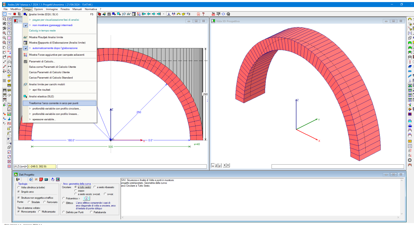
Fig. 1.4.1. Generazione di un arco per punti a partire da un arco circolare
