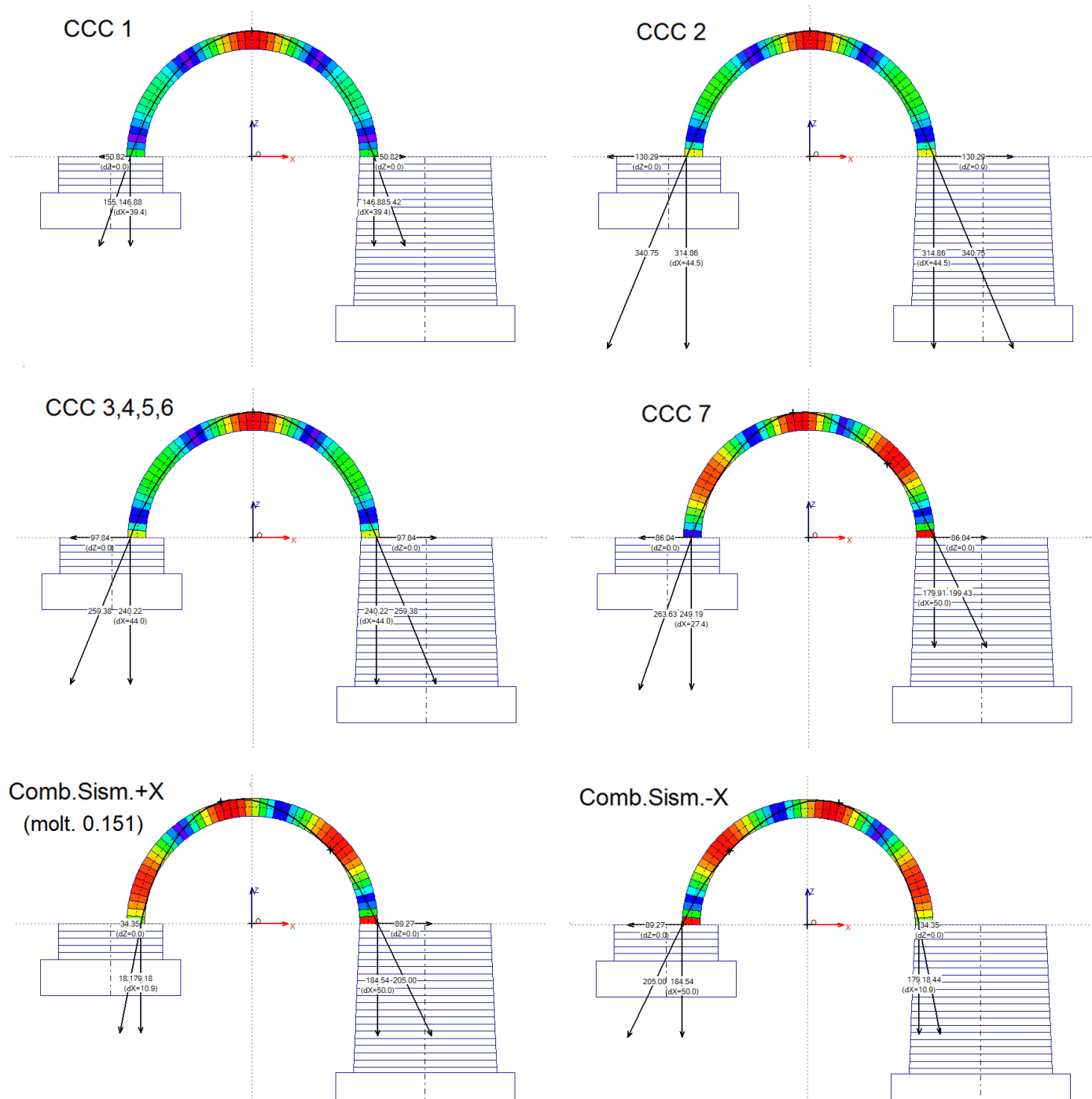
Fig. 2.3.10. Spinte alle imposte nella fase 1 per la campata SX
