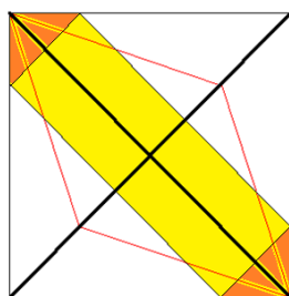
Fig. 1.3.7. Arco diagonale e zone in prossimità degli appoggi
