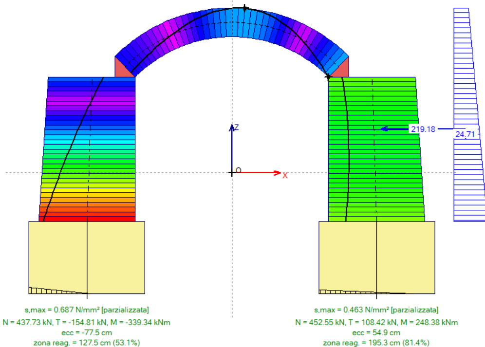
Fig. 2.1.38. Risultati Stato Attuale, Analisi Sismica -X. Curva delle pressioni
