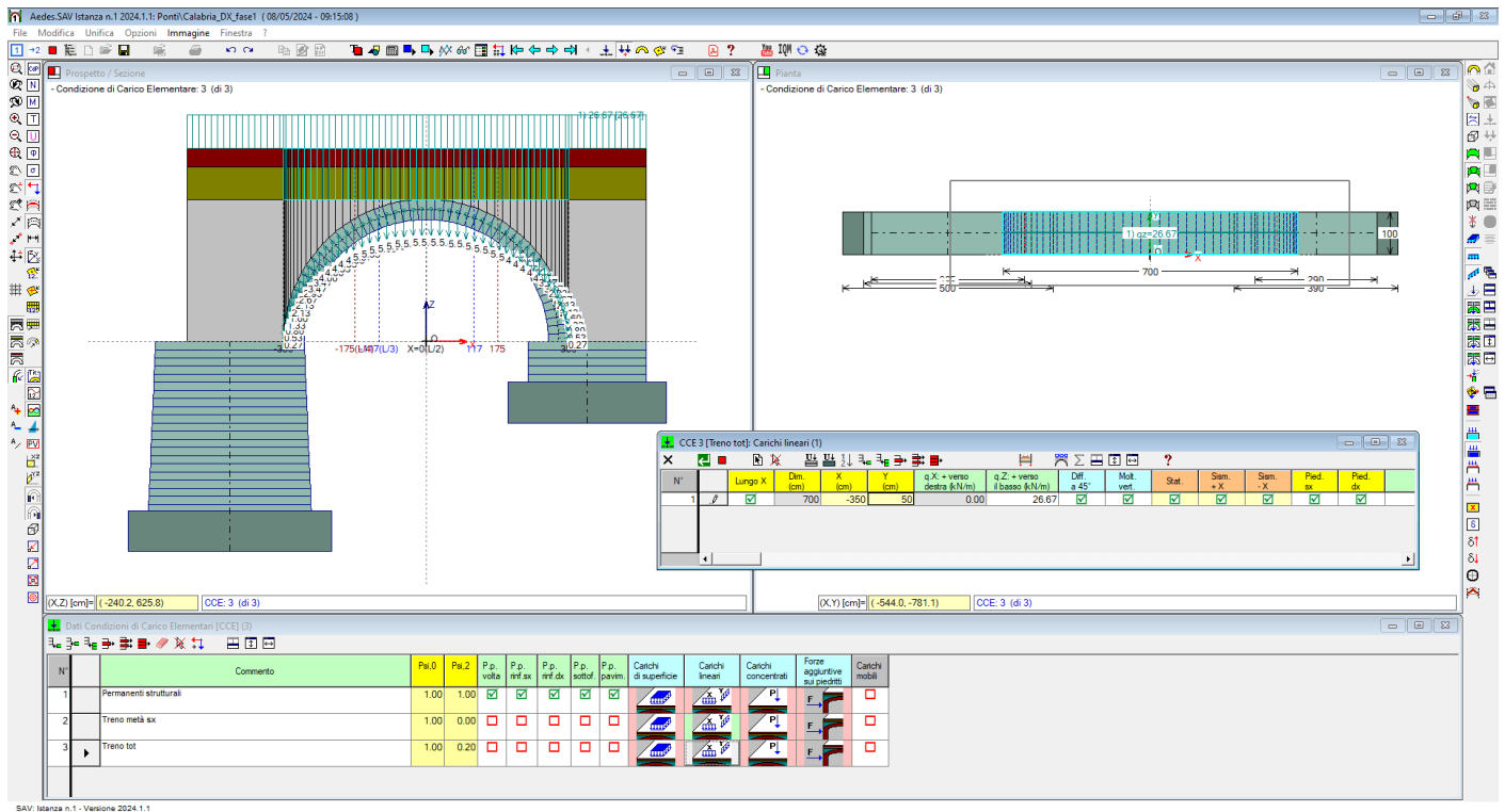
Fig. 2.3.19. Campata DX, CCE n°3, con carico da traffico ferroviario su tutto il ponte
