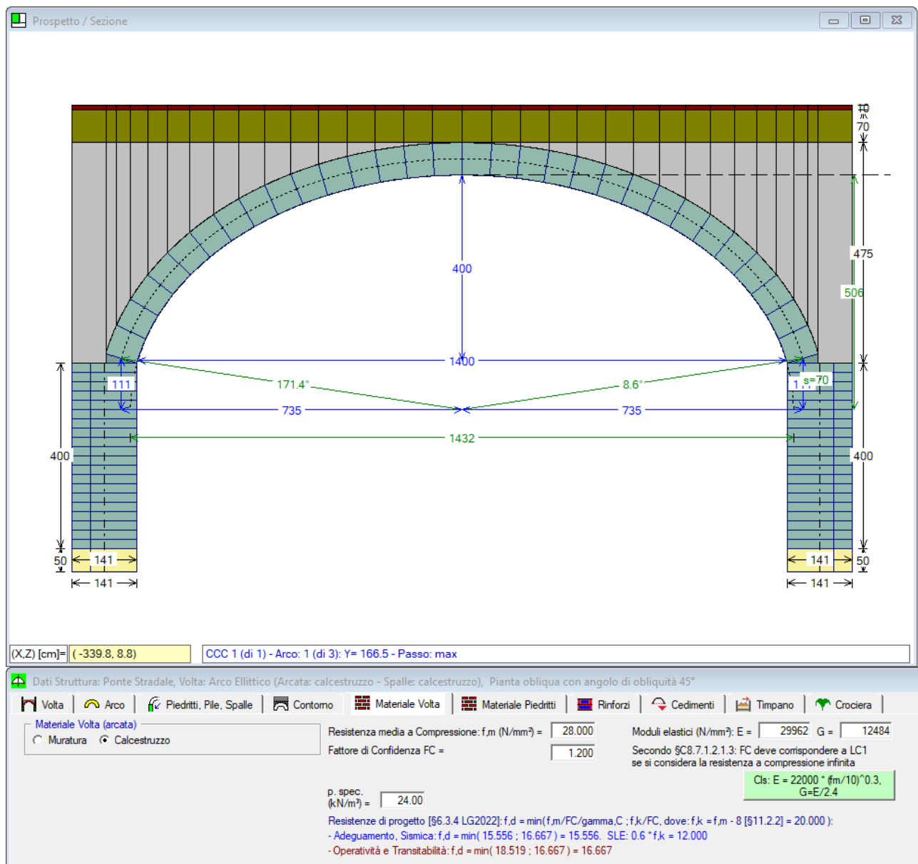
Fig. 2.4.19. Materiale Calcestruzzo C20/25
