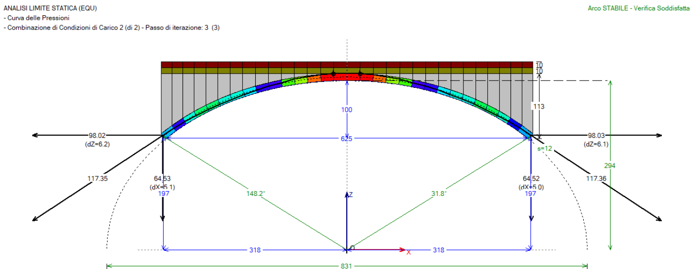
Fig. 1.3.10. Risultati analisi statica per l'arco diagonale. In evidenza, le spinte alle imposte
