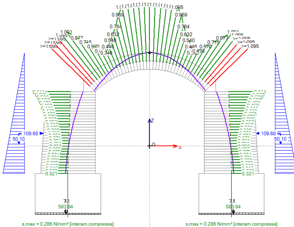
Fig. 2.1.34. Risultati Stato Attuale, Analisi Statica, CCC 3. Tensioni di Compressione
