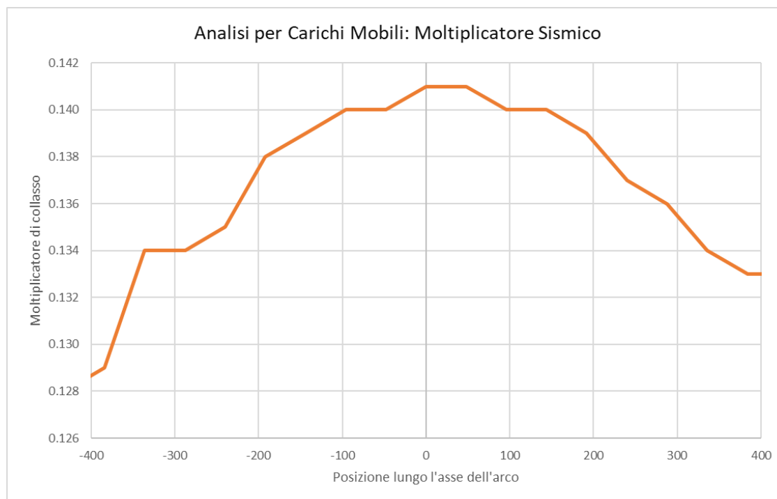
Fig. 4.3.8. Grafico dei risultati per il moltiplicatore sismico
