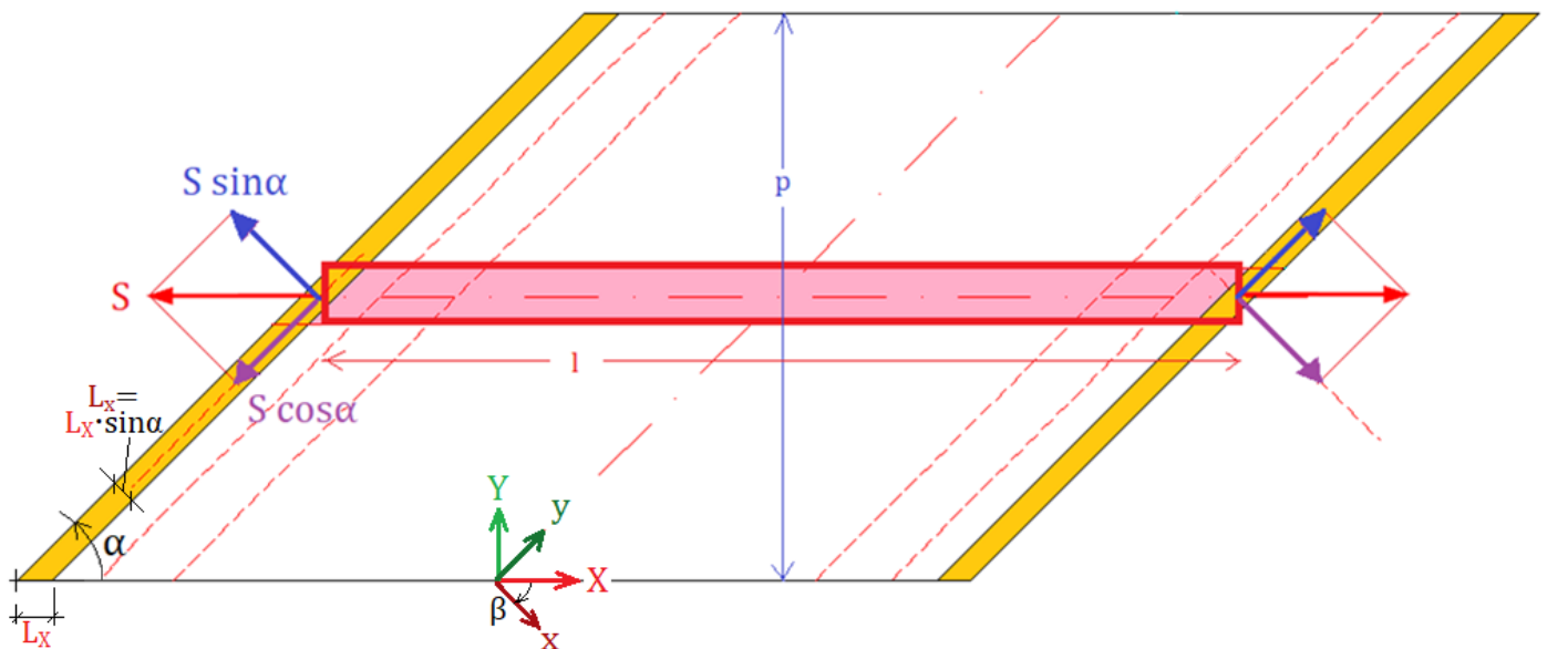
Fig. 2.4.3. Spinta trasmessa dalla volta ai piedritti: componenti nel piano e fuori piano
