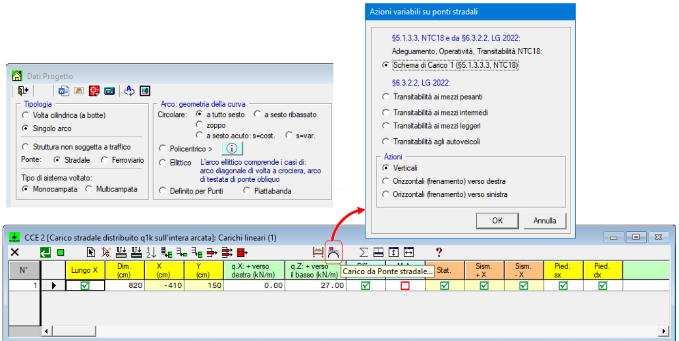
Fig. 2.5.1. Inserimento dei carichi stradali
