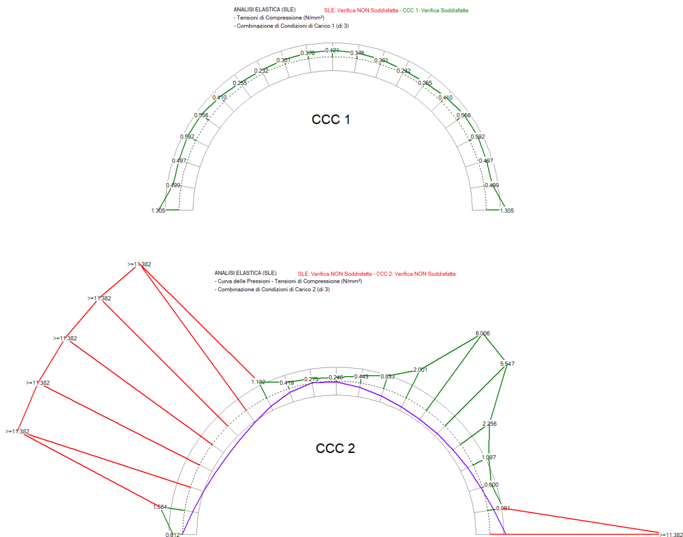
Fig. 3.4.5. Curva delle pressioni e Tensioni di compressione per le CCC 1 e 2
