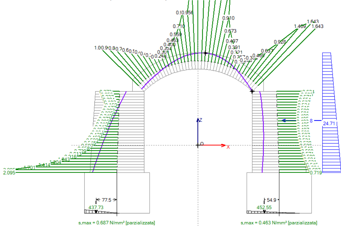
Fig. 2.1.39. Risultati Stato Attuale, Analisi Sismica -X. Tensioni di Compressione
