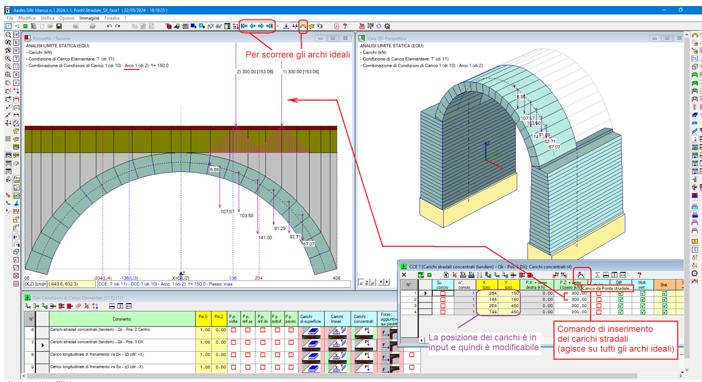
Fig. 2.3.43. Carichi concentrati stradali
