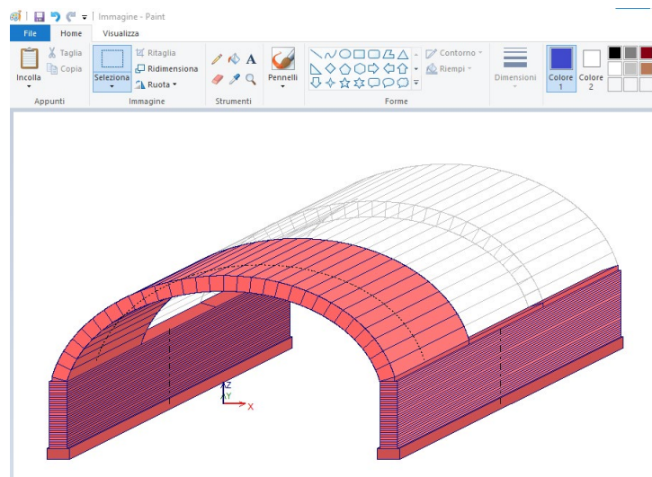
Fig. 2.4.16. Vista 3D con limiti imposti
