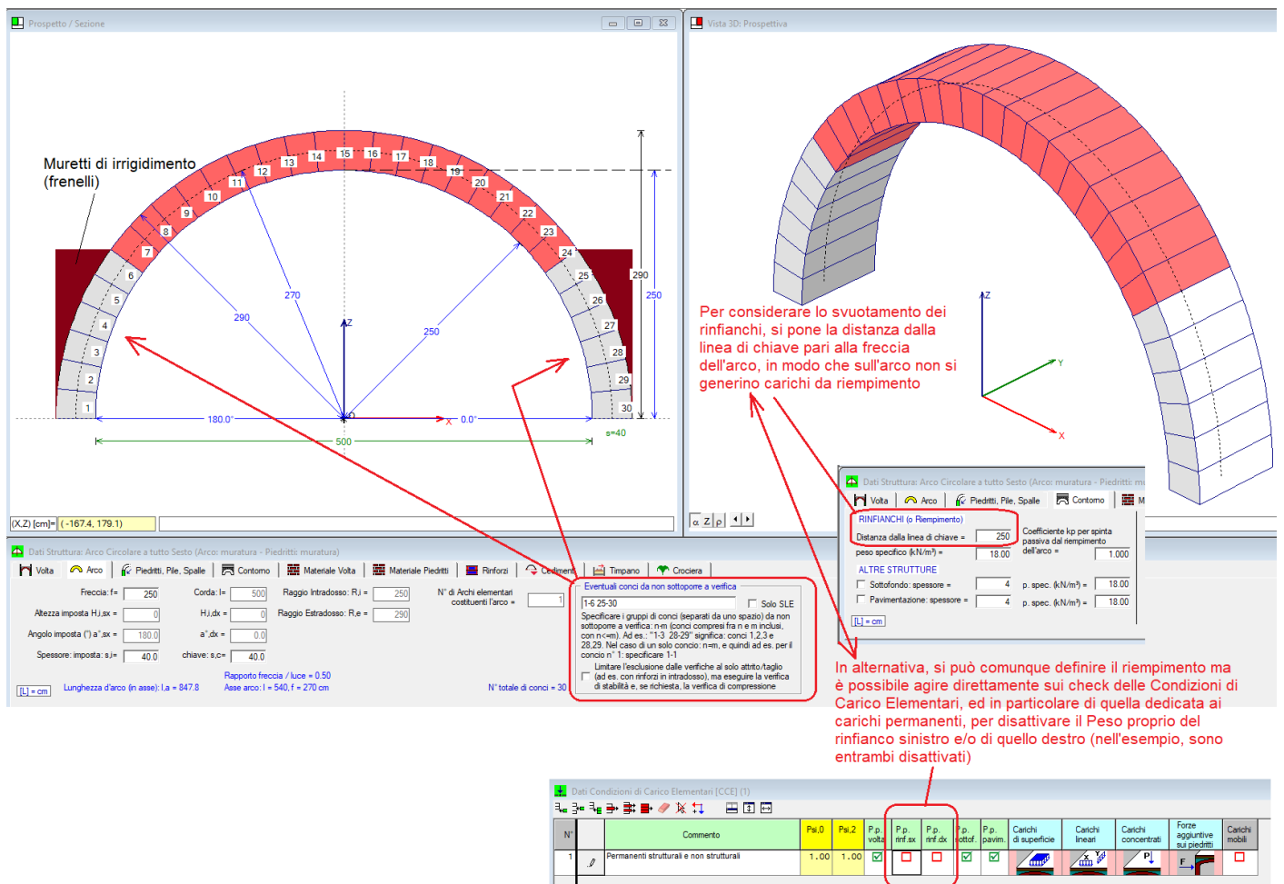
Fig. 1.6.3.2. Irrigidimento dei conci alle imposte e modellazione dello svuotamento dei rinfianchi
