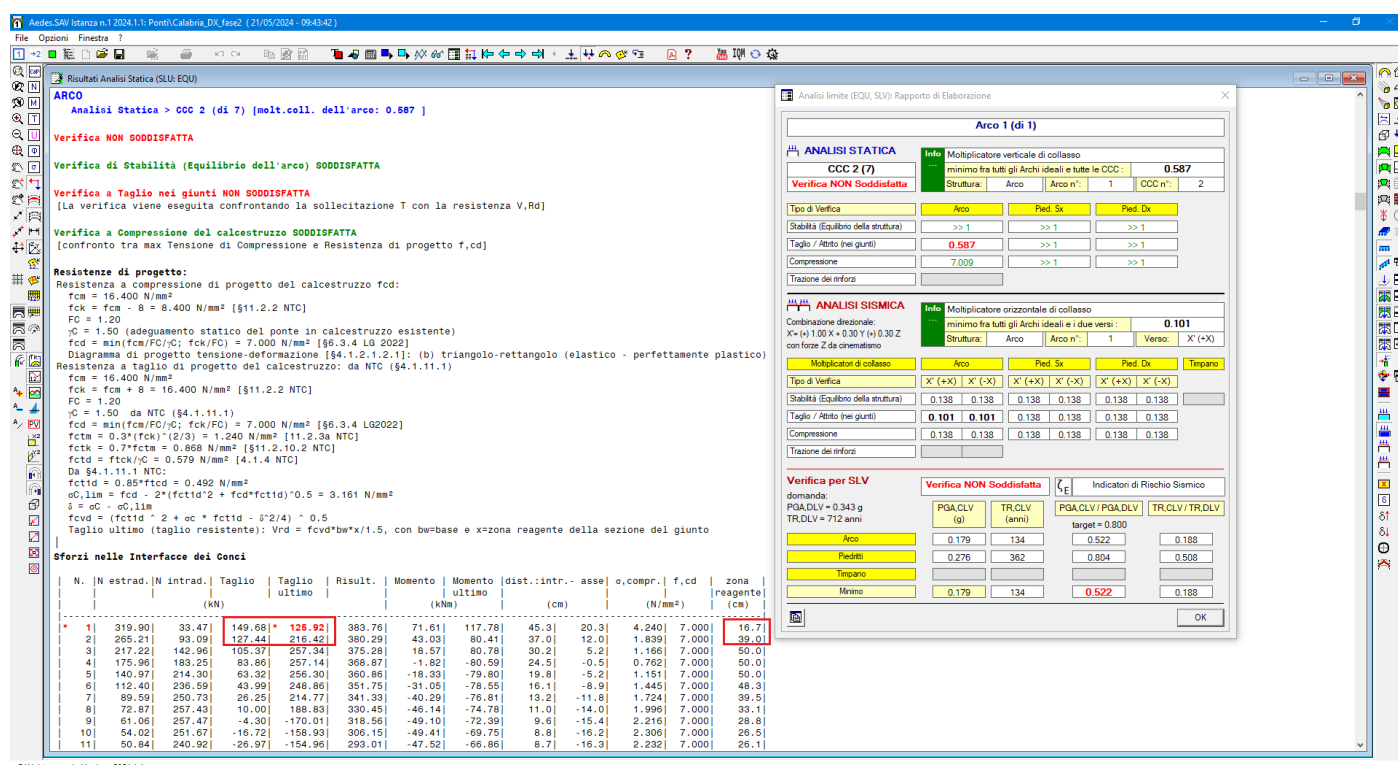
Fig. 2.3.34. Campata destra: verifica a taglio in corrispondenza dell'imposta
