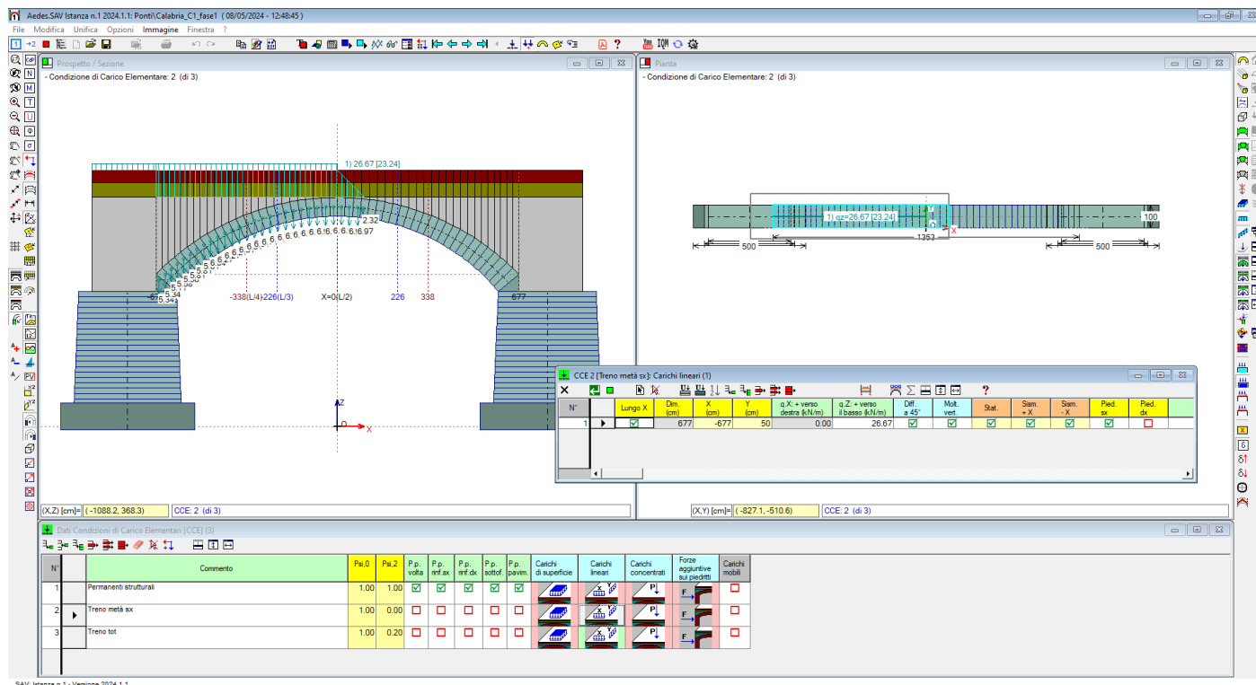
Fig. 2.3.13. Campata C1, CCE n°2, con carico da traffico ferroviario su metà campata
