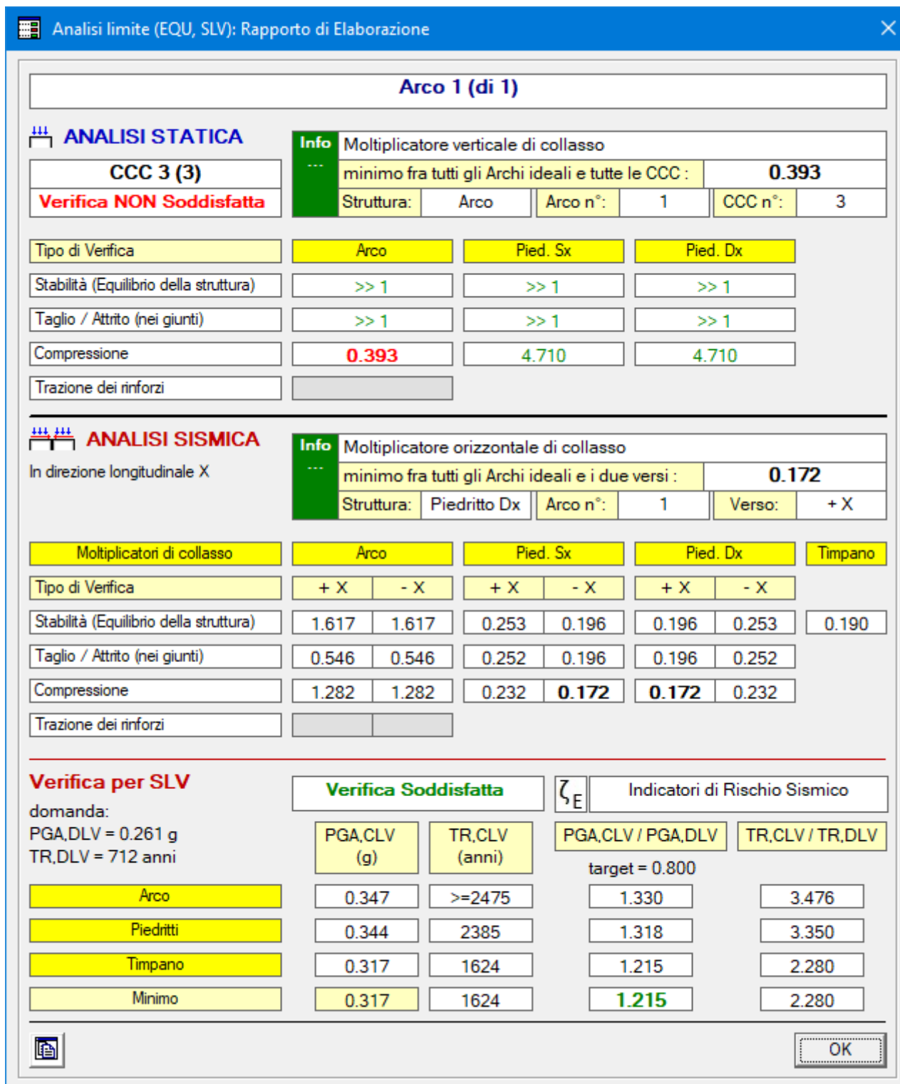
Fig. 2.1.35. Risultati Stato Attuale, Analisi Statica, CCC 2 e Analisi Sismica. Report dei moltiplicatori di collasso
