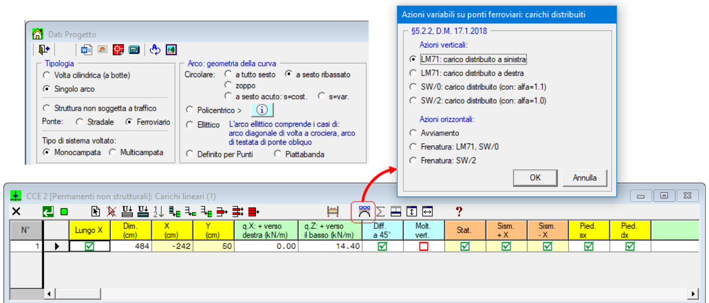
Fig. 2.5.2. Inserimento dei carichi ferroviari
