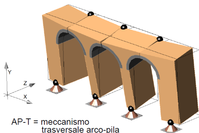
Fig. 2.3.70. Meccanismo trasversale arco-pila (da [1])
