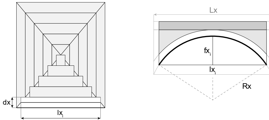
Fig. 1.3.4. Volta a crociera: (a) in pianta, discretizzazione in lunette; (b) in sezione, lunetta in direzione x
