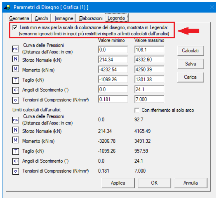
Fig. 2.3.61. Limiti per i risultati coerenti per tutti i modelli del ponte multicampata
