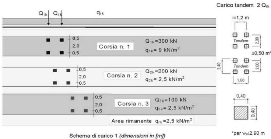
Fig. 2.5.3. Schemi di carico su ponte stradale secondo D.M. 17.1.2018
