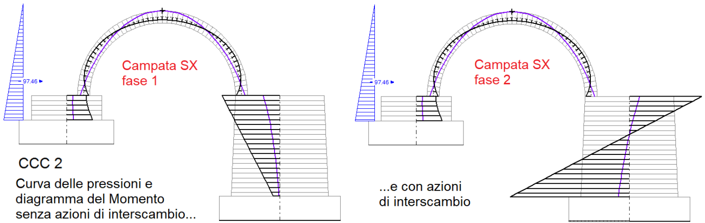
Fig. 2.3.29. Diagramma dei momenti e Curva delle pressioni per la CCC statica n°2
