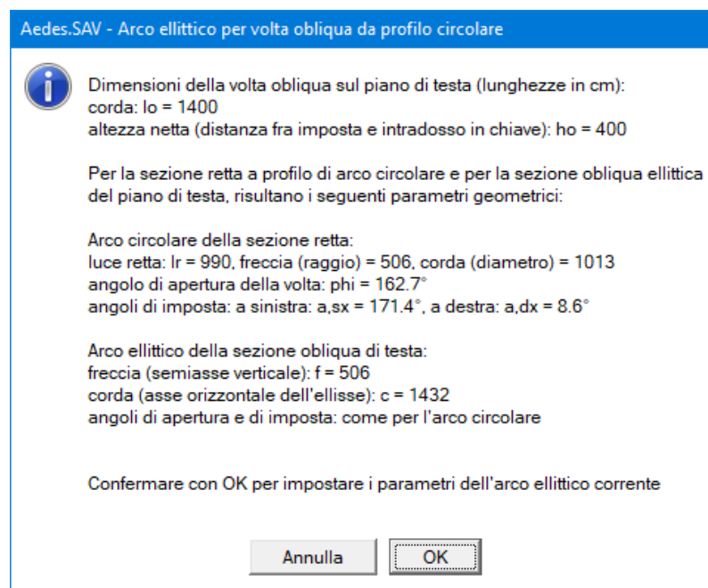
Fig. 2.4.12. Predisposizione automatica dei dati geometrici della volta obliqua
