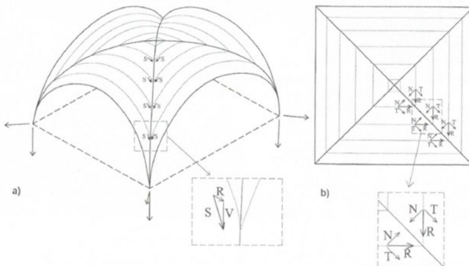
Figura 2.50. Volta a crociera con schematizzazione delle azioni trasferite dagli archi, che idealmente costituiscono la volta, all'arcone diagonale
