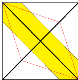
Fig. 1.3.6. Ingombro in pianta dell'arco diagonale
