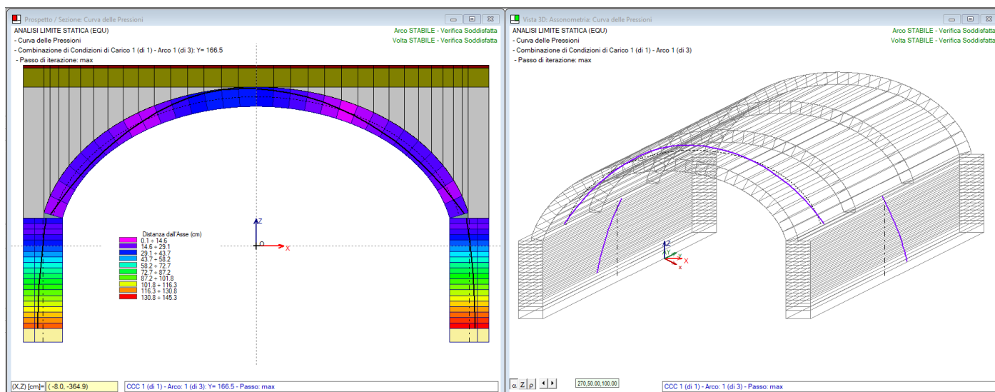
Fig. 2.4.25. Curva delle pressioni in vista 3D
