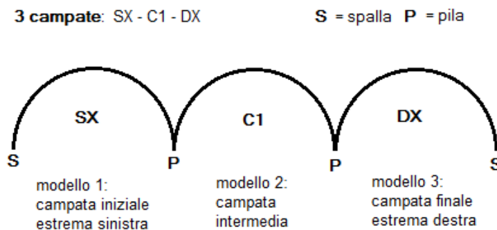
Fig. 2.3.9. Modelli del ponte a 3 campate
