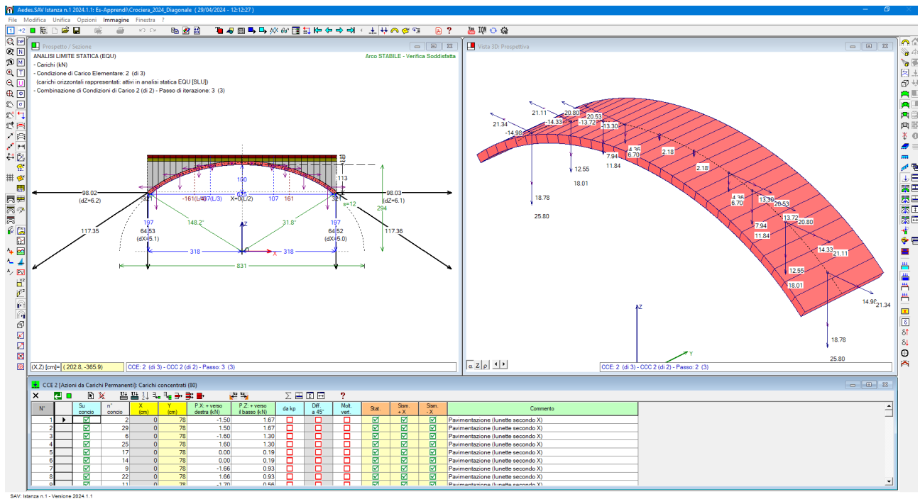
Fig. 1.3.9. Azioni concentrate applicate dalle lunette sull'arco diagonale
