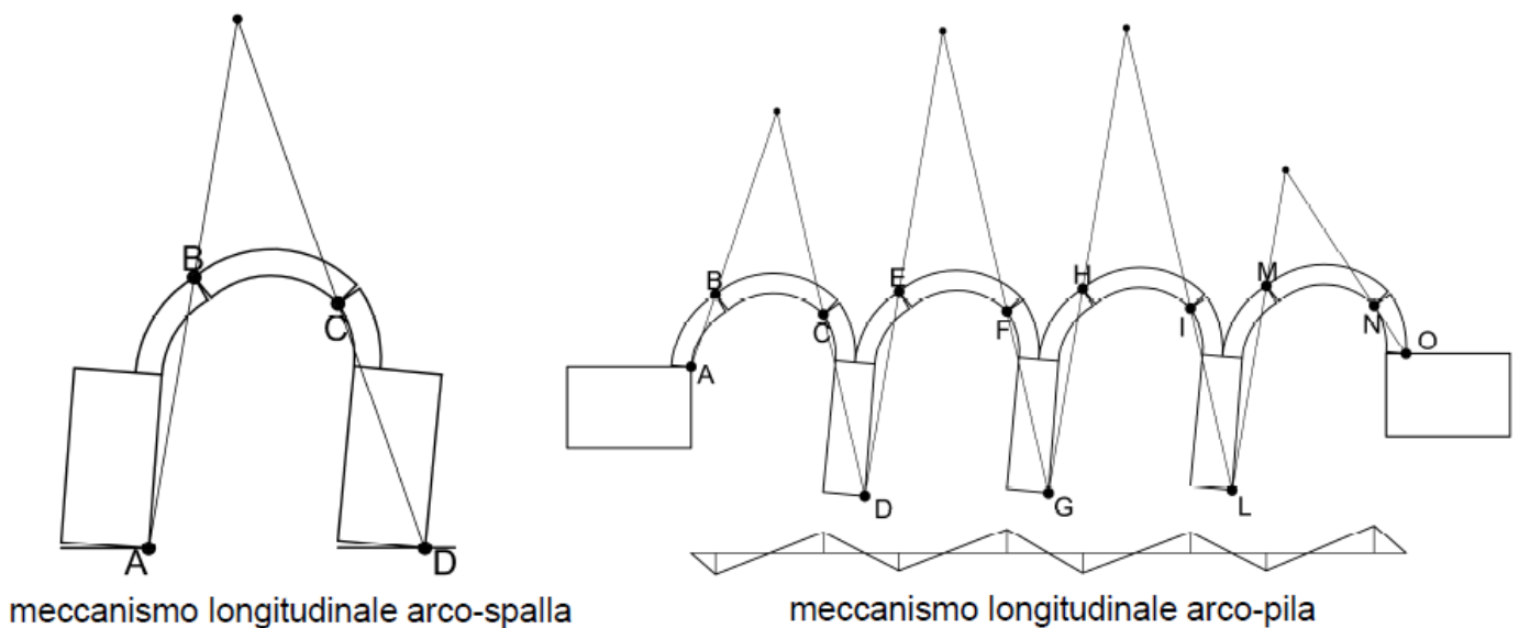
Fig. 2.3.69. Meccanismi globali longitudinali (da [1])
