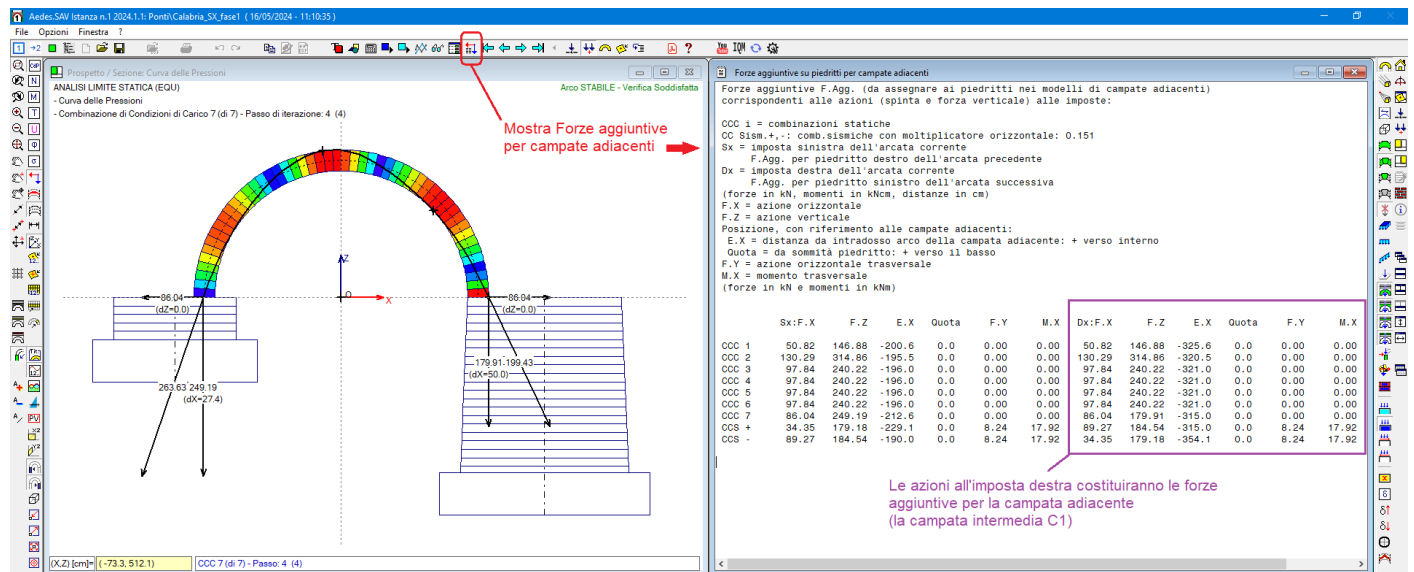
Fig. 2.3.11. Campata SX: quadro riepilogativo forze alle imposte (aggiuntive per la campata C1)
