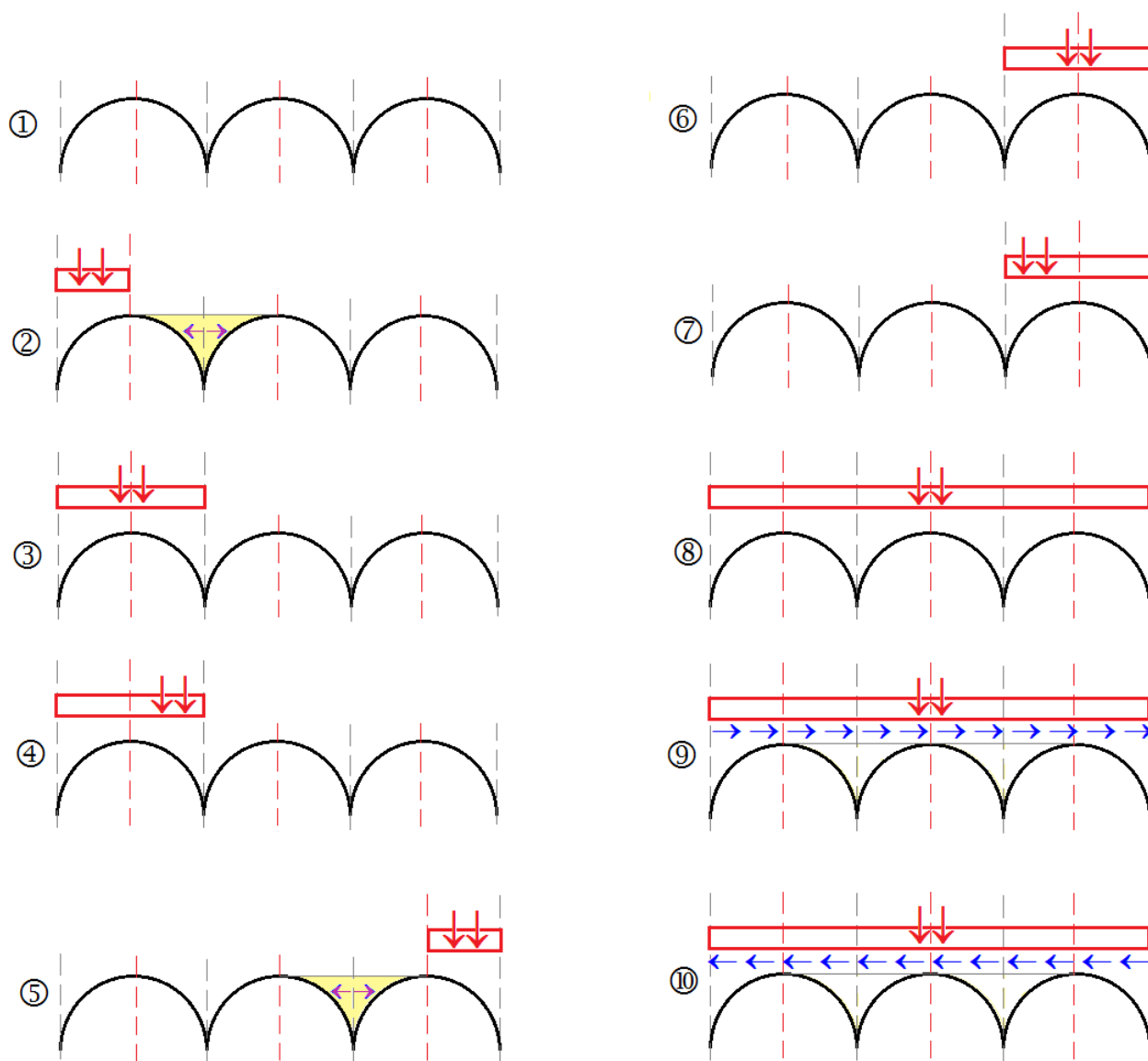
Fig. 2.3.42. Combinazioni di Condizioni di Carico
