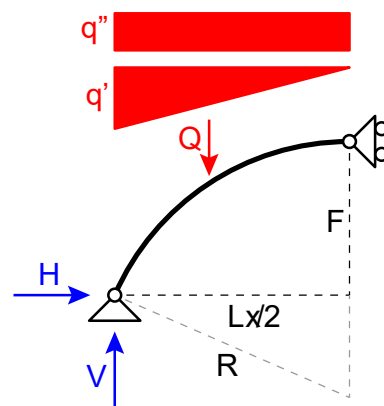
Fig. 1.3.5. Arco circolare: schema statico per il calcolo delle azioni d'imposta (spinta e forza verticale)
