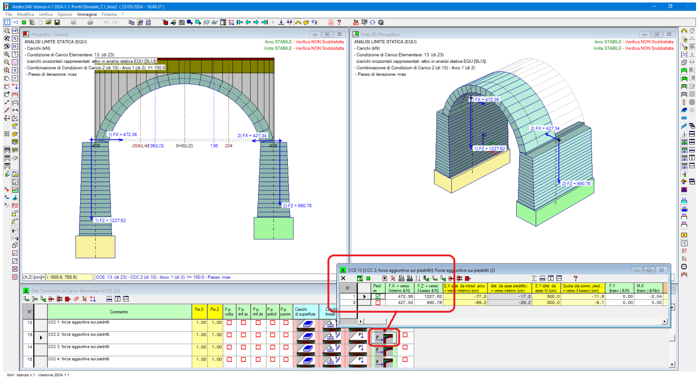
Fig. 2.3.56. Campata intermedia: azioni di interscambio provenienti dalle campate sinistra e destra
