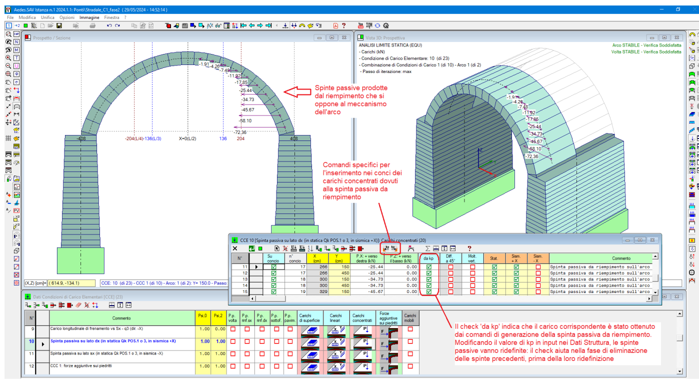
Fig. 2.3.75. Inserimento delle forze di spinta passiva
