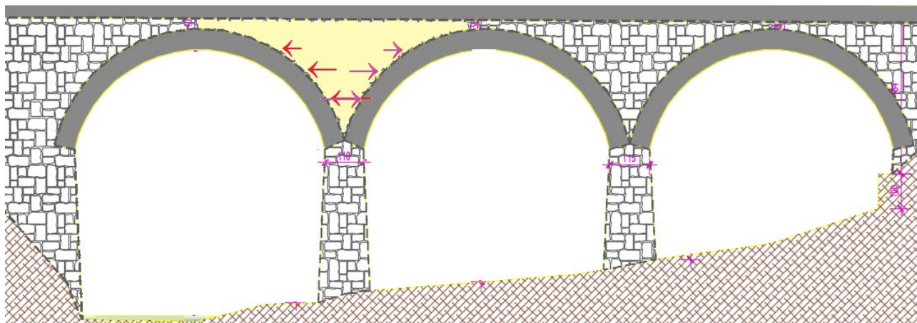
Fig. 2.3.41. Spinte passive sviluppate nei rinfianchi
