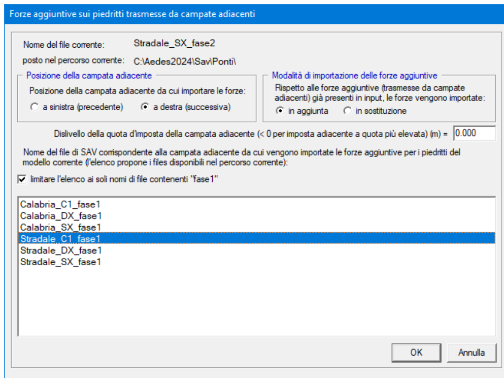
Fig. 2.3.49. Campata sinistra: importazione delle azioni di interscambio provenienti dalla campata intermedia
