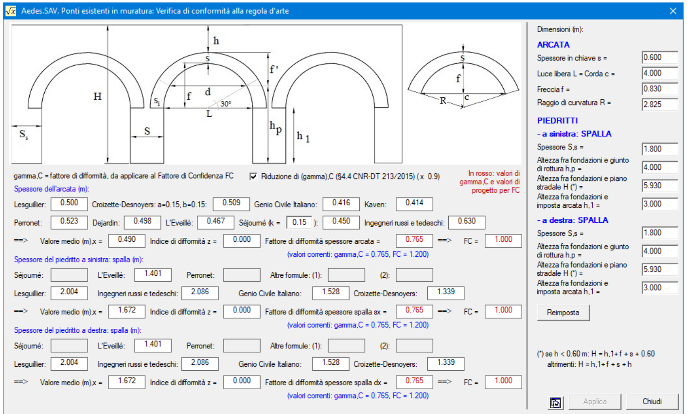
Fig. 2.1.7. Conformità alla regola dell'arte per le strutture dei ponti in muratura
