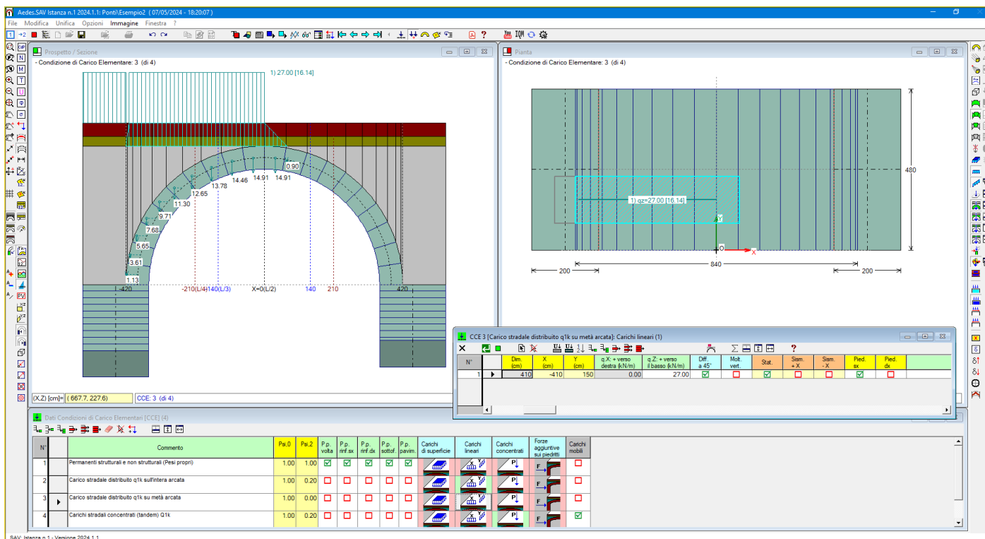
Fig. 2.2.8. Carichi della CCE 3
