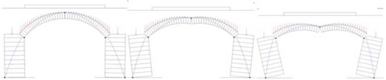
Fig. 2.1.10. Movimento dei piedritti verso l'esterno, sotto l'azione delle spinte alle imposte dell'arco
