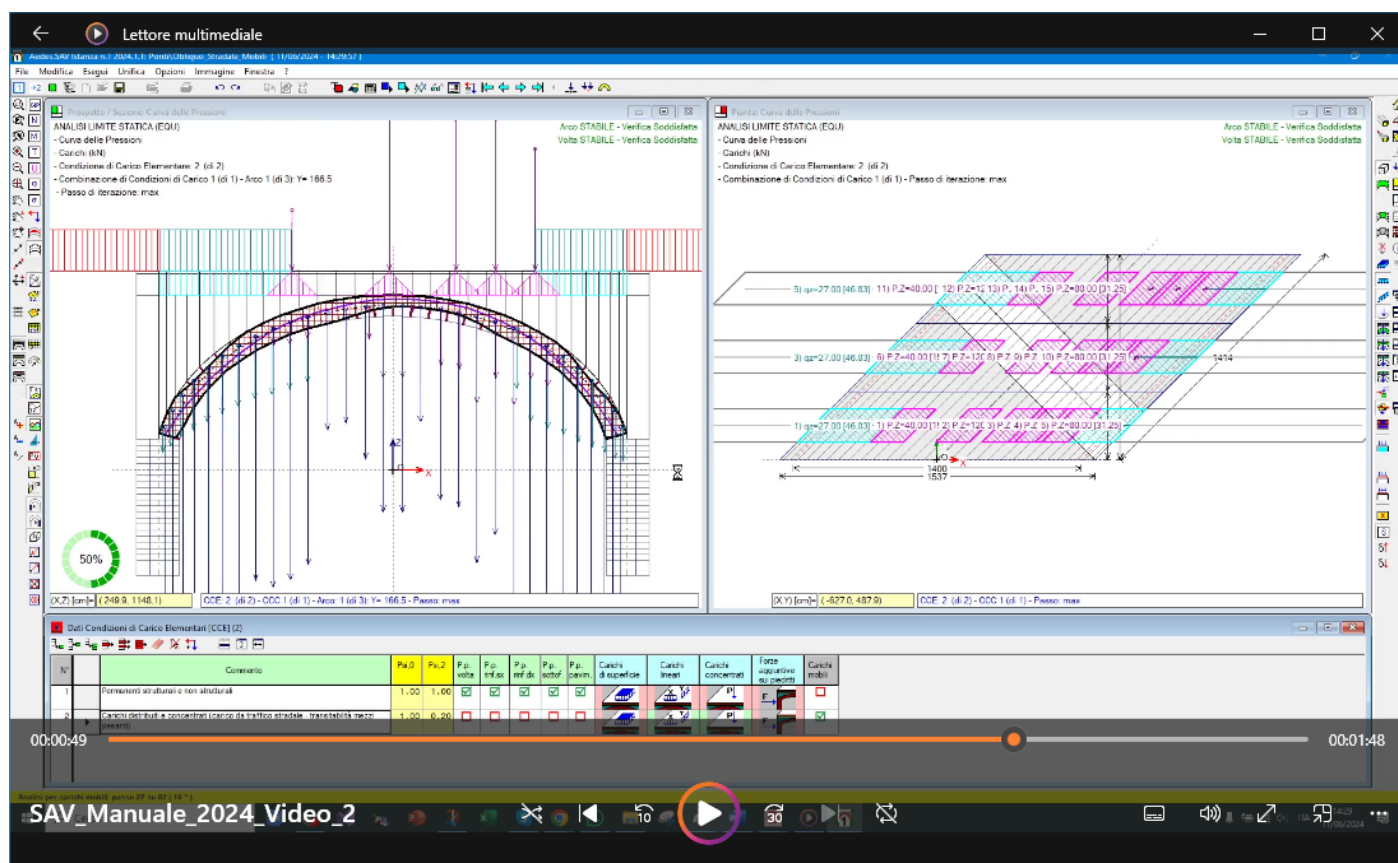
Fig. 2.4.23. Video con analisi per carichi mobili
