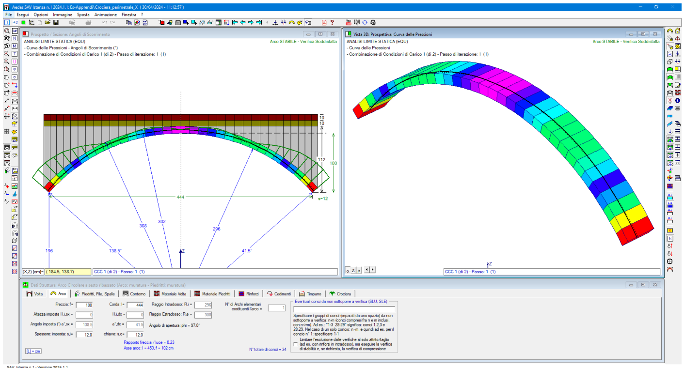
Fig. 1.3.11. Risultati analisi statica per un arco perimetrale
