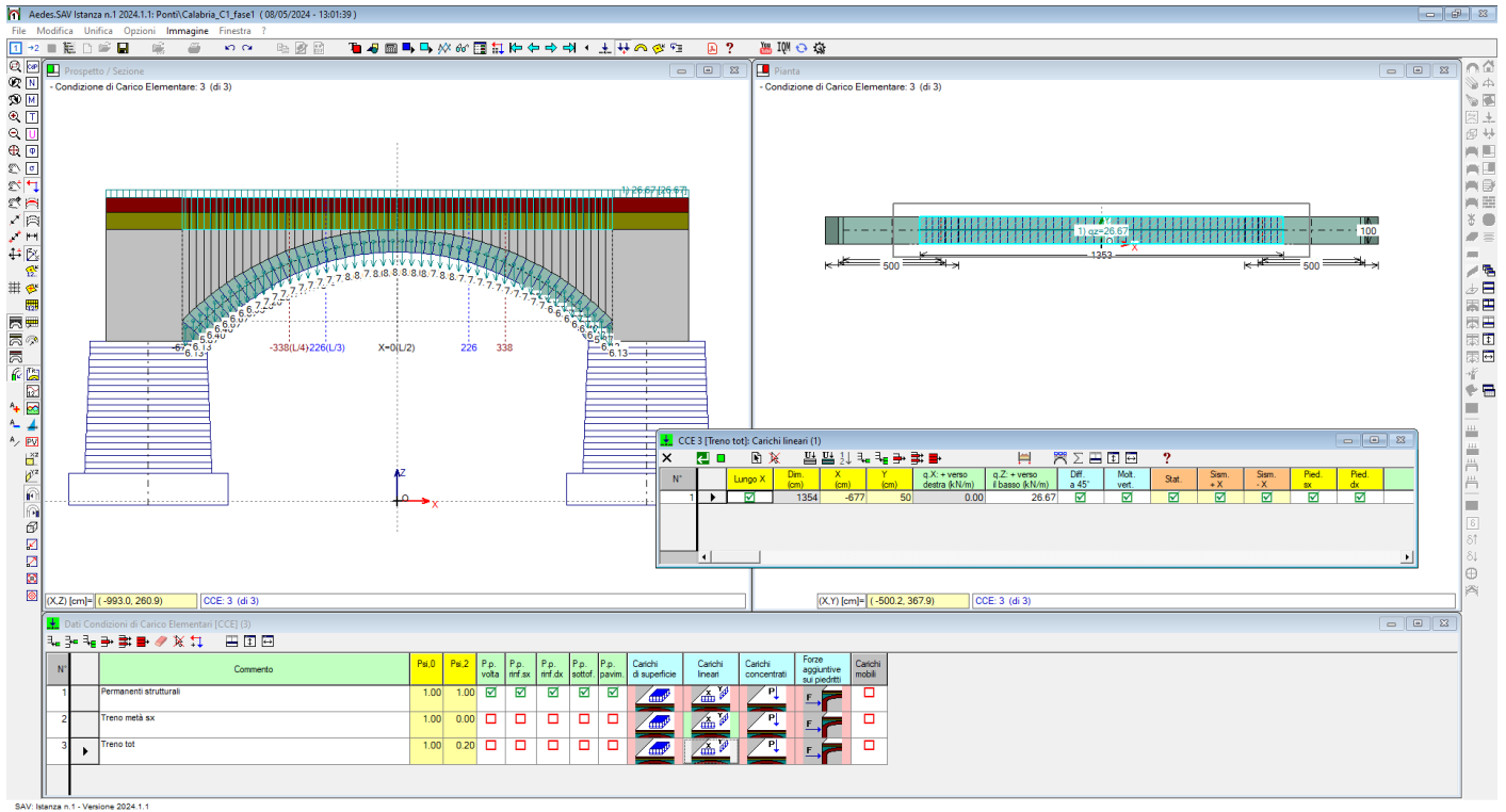
Fig. 2.3.14. Campata C1, CCE n°3, con carico da traffico ferroviario su tutto il ponte
