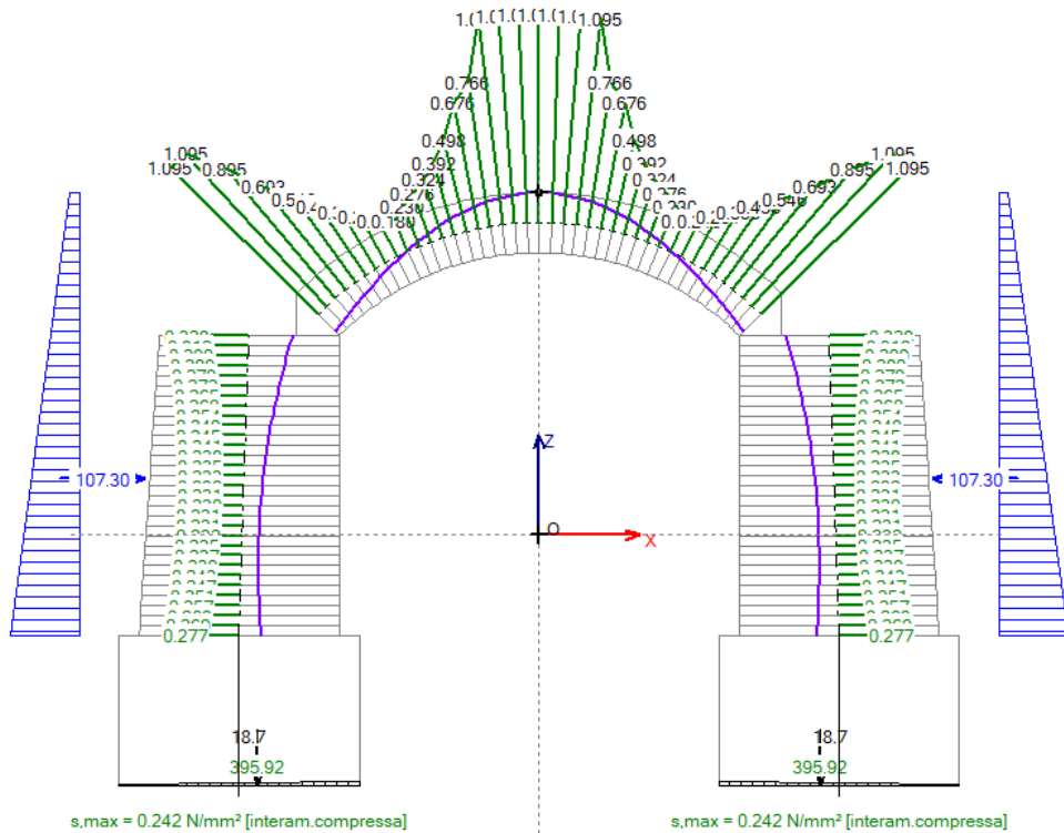
Fig. 2.1.28. Risultati Stato Attuale, Analisi Statica, CCC 1. Tensioni di Compressione
