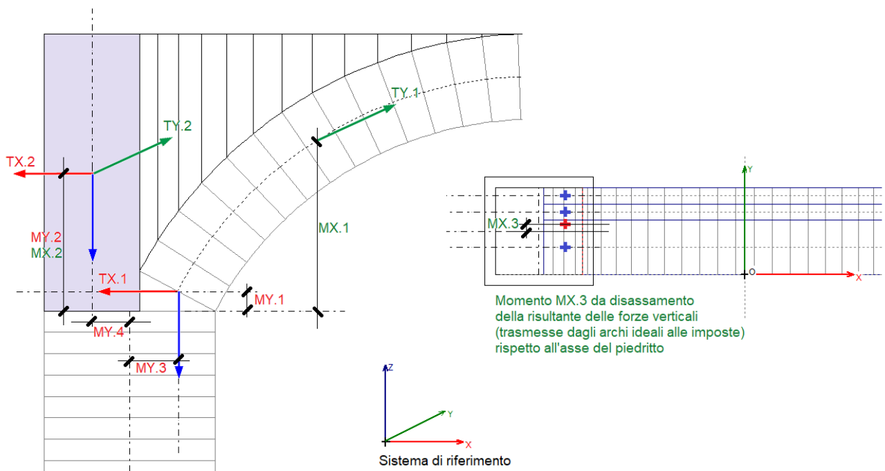
Fig. 1.2.2. Azioni longitudinali e trasversali sui piedritti
