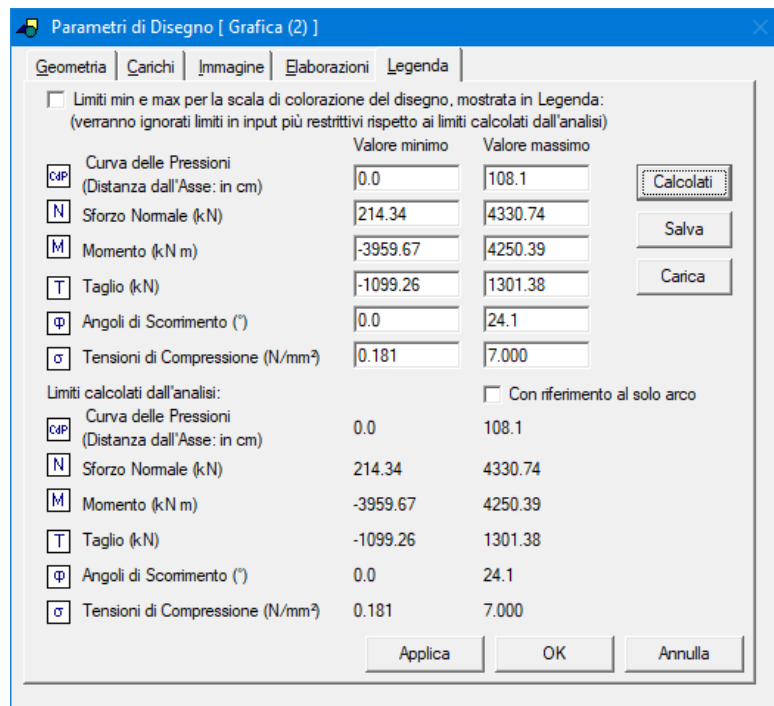
Fig. 2.3.60. Scheda Legenda della finestra Parametri di Disegno
