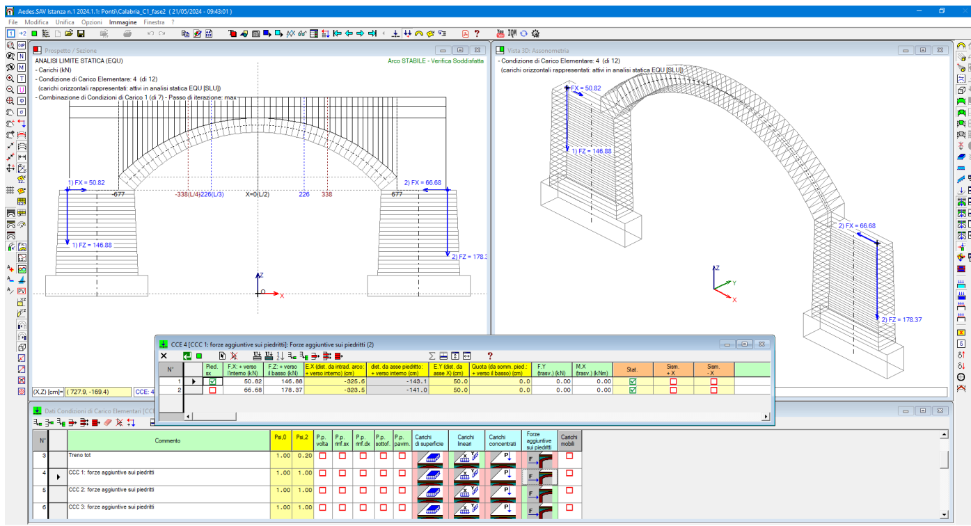
Fig. 2.3.31. Campata C1: azioni di interscambio dalle campate adiacenti, con focus sulla CCE n°4
