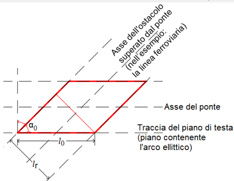
Fig. 2.4.9. Definizione della volta per il ponte obliquo
