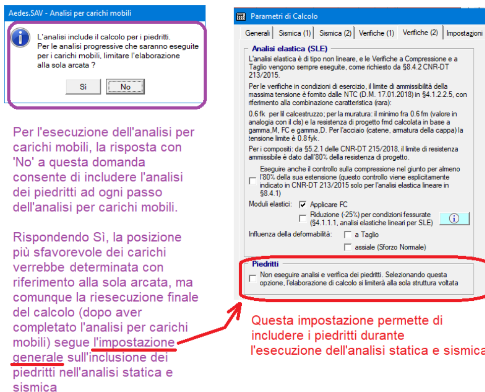
Fig. 4.3.1. Analisi per carichi mobili, considerando o meno il contributo dei piedritti
