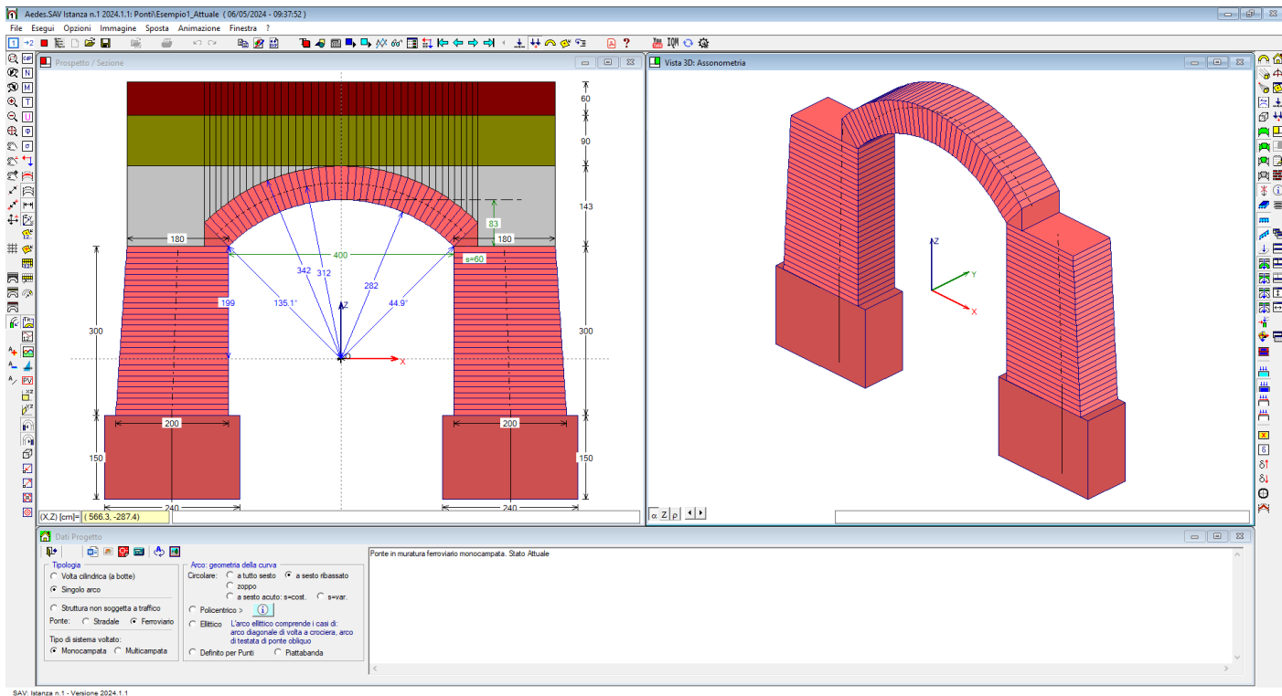
Fig. 2.1.4. Stato Attuale: Dati Progetto
