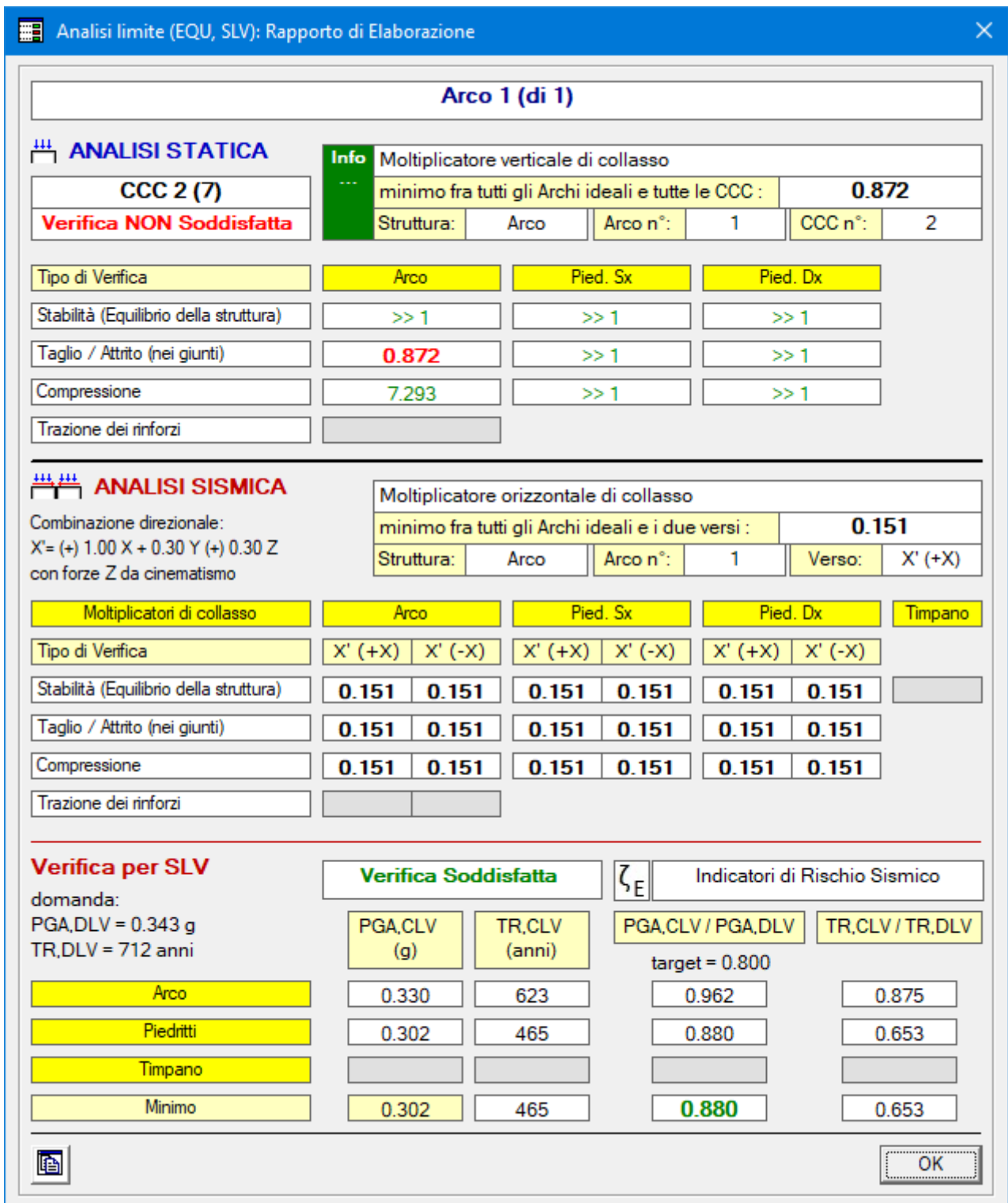
Fig. 2.3.28. Campata SX: risultati definitivi (fase 2)
