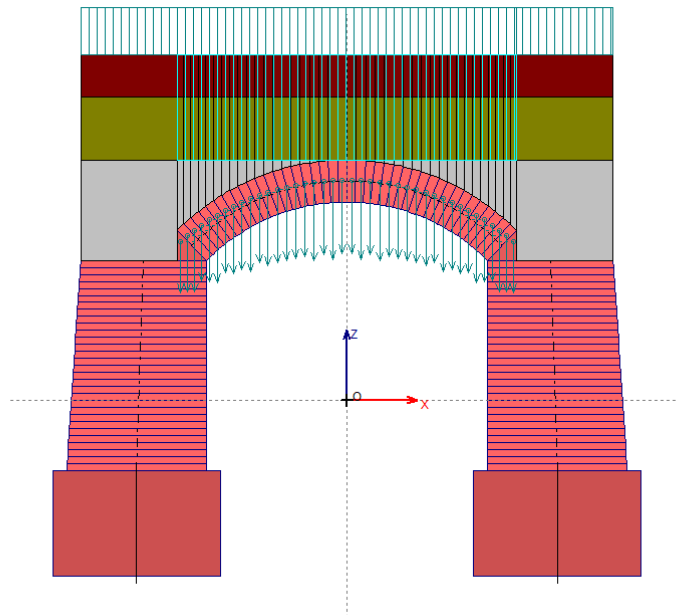
Fig. 2.1.25. Carichi per CCE n.4
