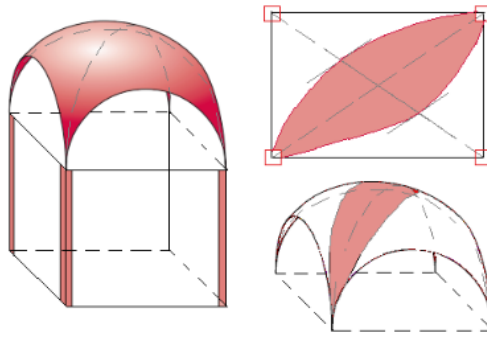
Fig. 1.4.7. Individuazione dell'arco diagonale nella volta a vela
