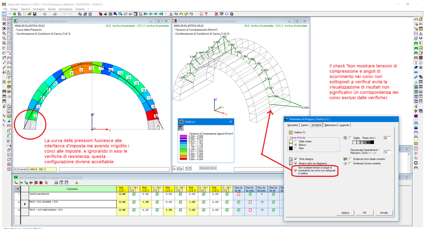
Fig. 3.4.9. Risultati per la CCC 2 nel caso di conci alle imposte irrigiditi
