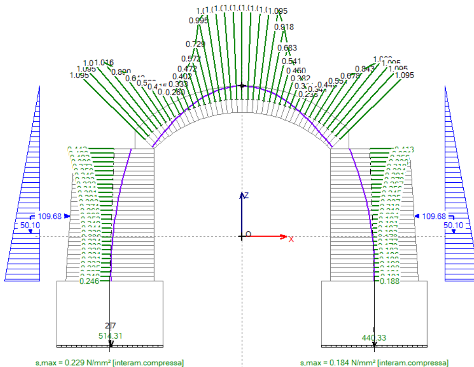
Fig. 2.1.31. Risultati Stato Attuale, Analisi Statica, CCC 2. Tensioni di Compressione
