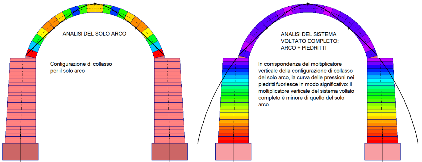
Fig. 4.1.3. Comportamento del sistema voltato completo diverso da quello del solo arco
