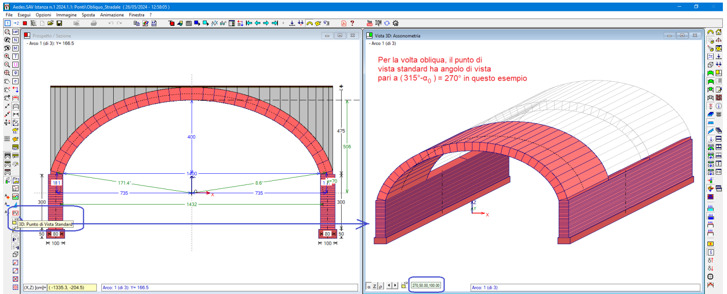
Fig. 2.4.15. Vista 3D con punto di vista standard per la volta obliqua
